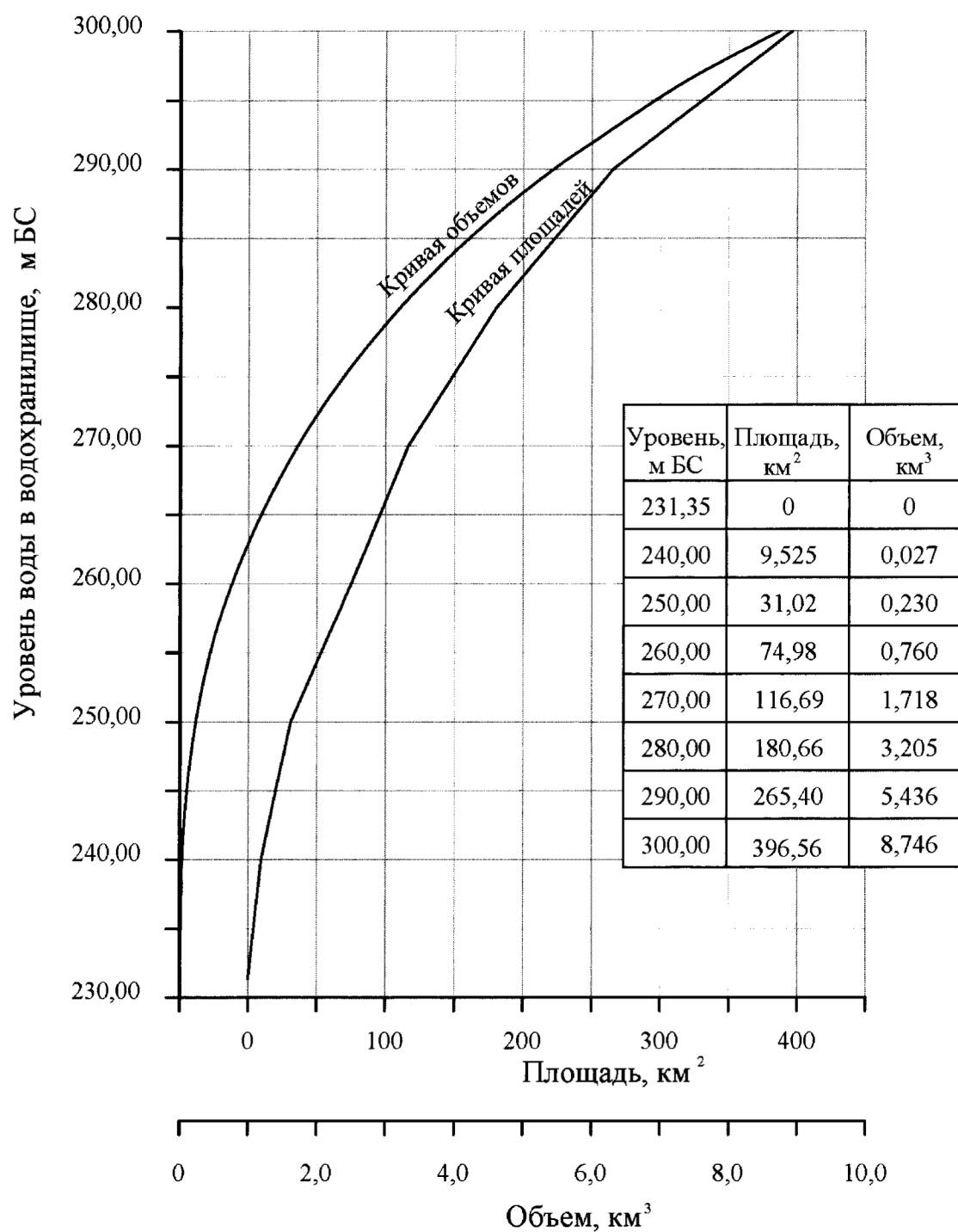
Статические кривые зависимости объема воды и площади зеркала Усть-Среднеканского водохранилища от уровня воды
