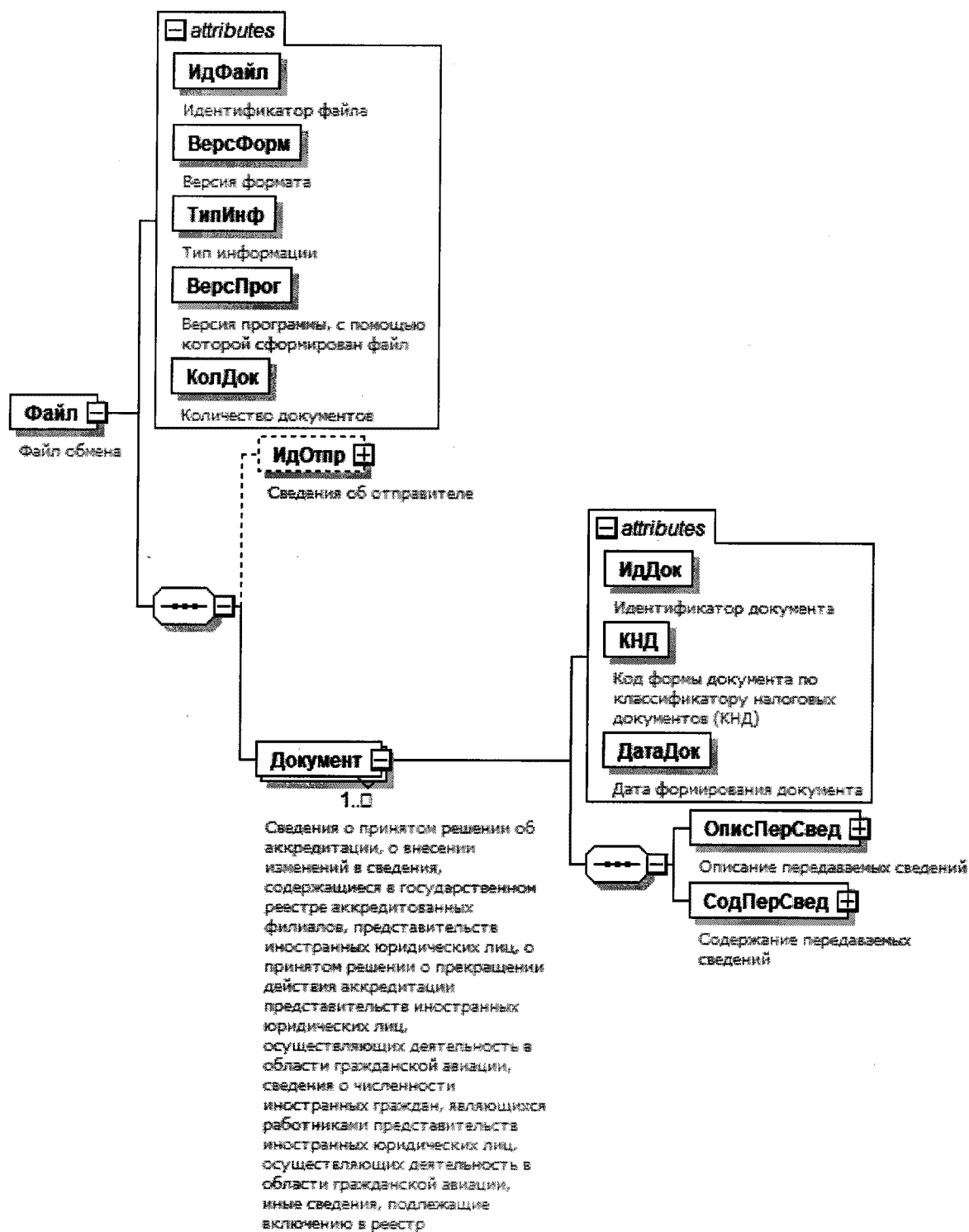
Рис.1. Диаграмма структуры файла обмена
