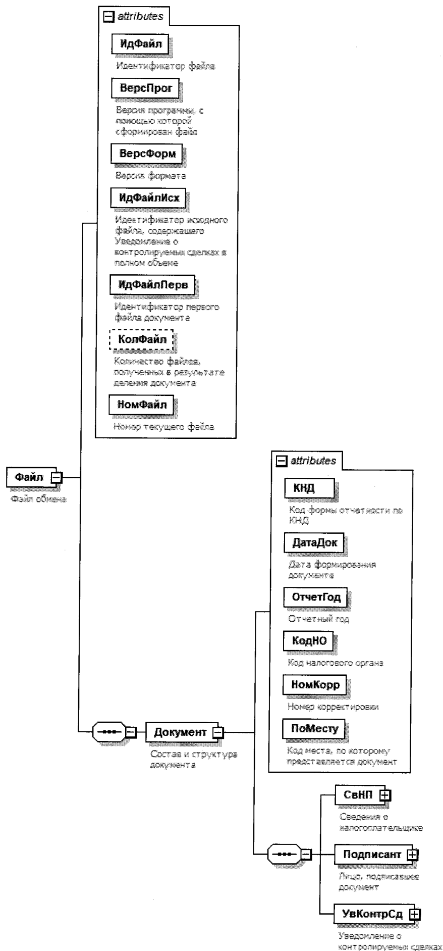
Рисунок 1. Диаграмма структуры файла обмена
