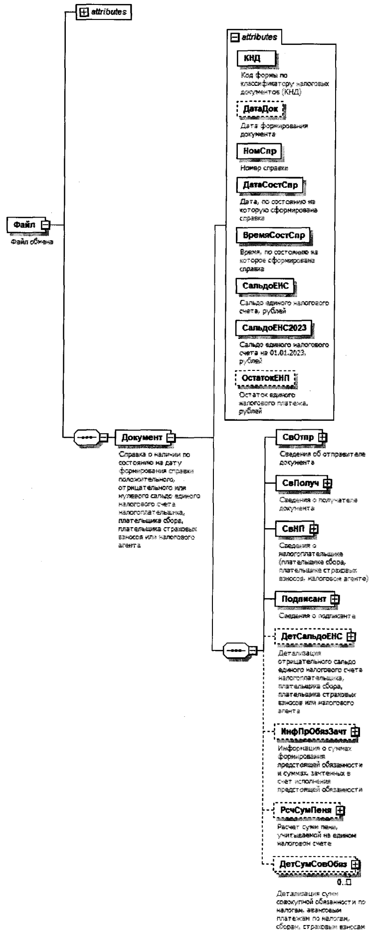
Рисунок 1. Диаграмма структуры файла обмена
