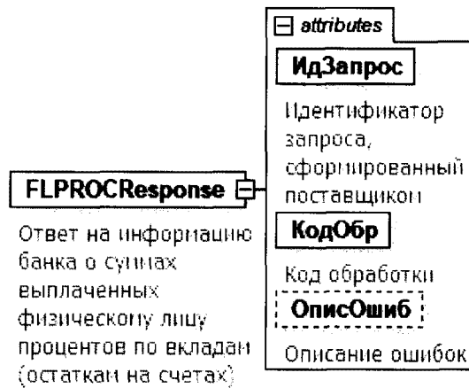
Рисунок 2. Диаграмма структуры файла обмена
