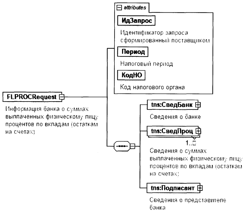
Рисунок 1. Диаграмма структуры документа
