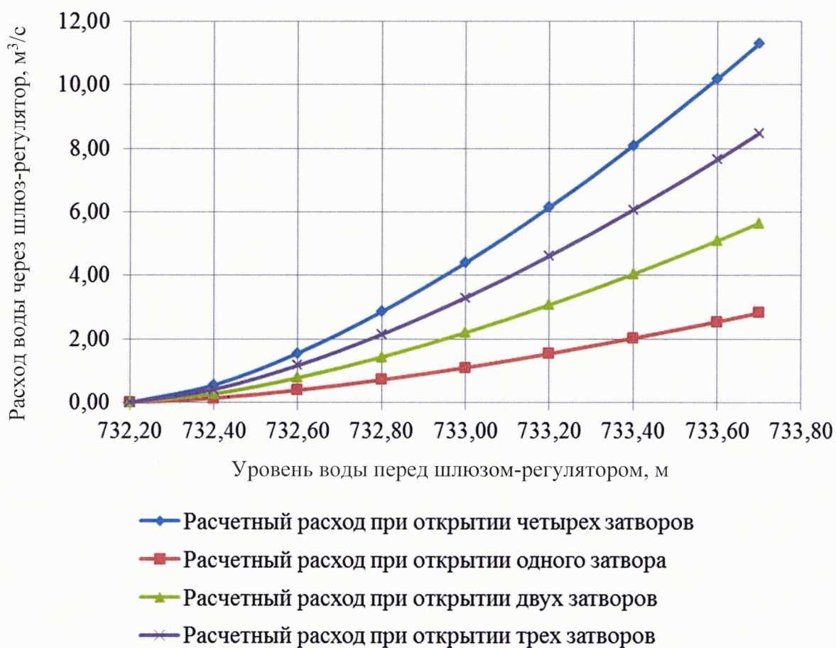
Пропускная способность шлюза-регулятора
