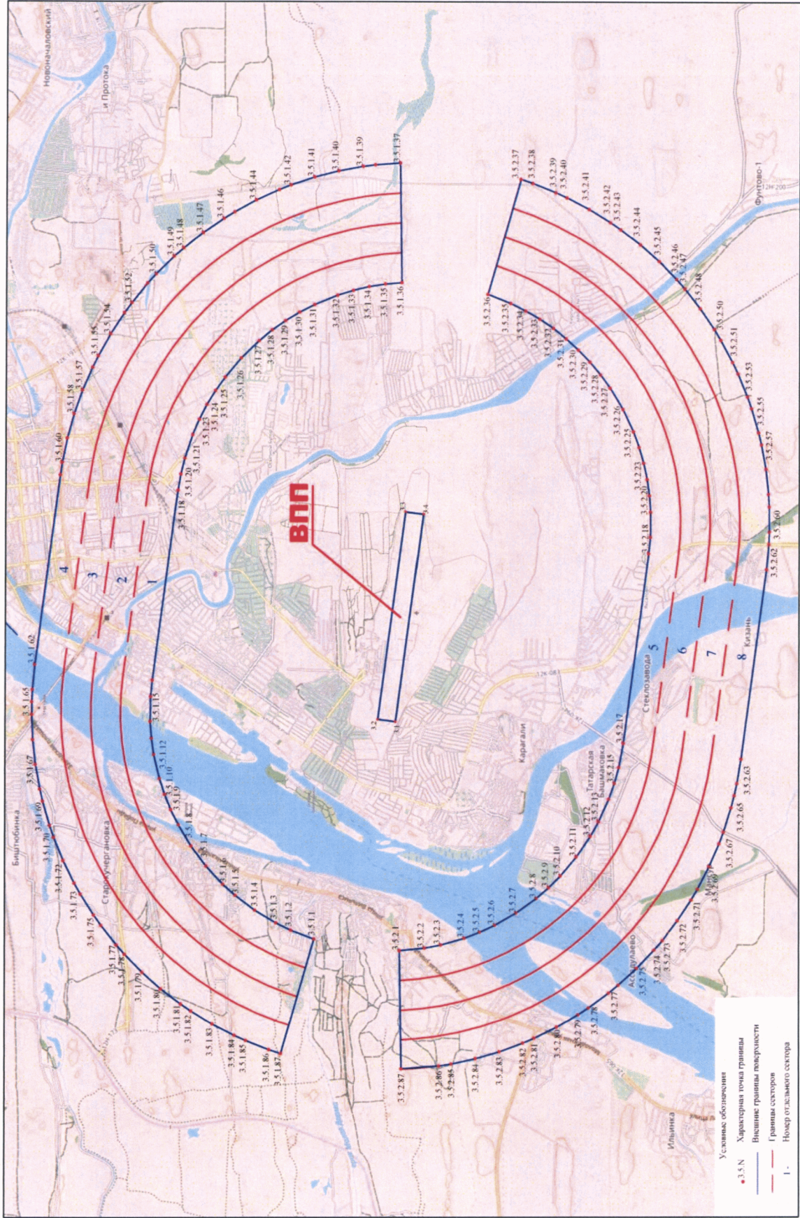
Схема 3.6 (Коническая поверхность)
