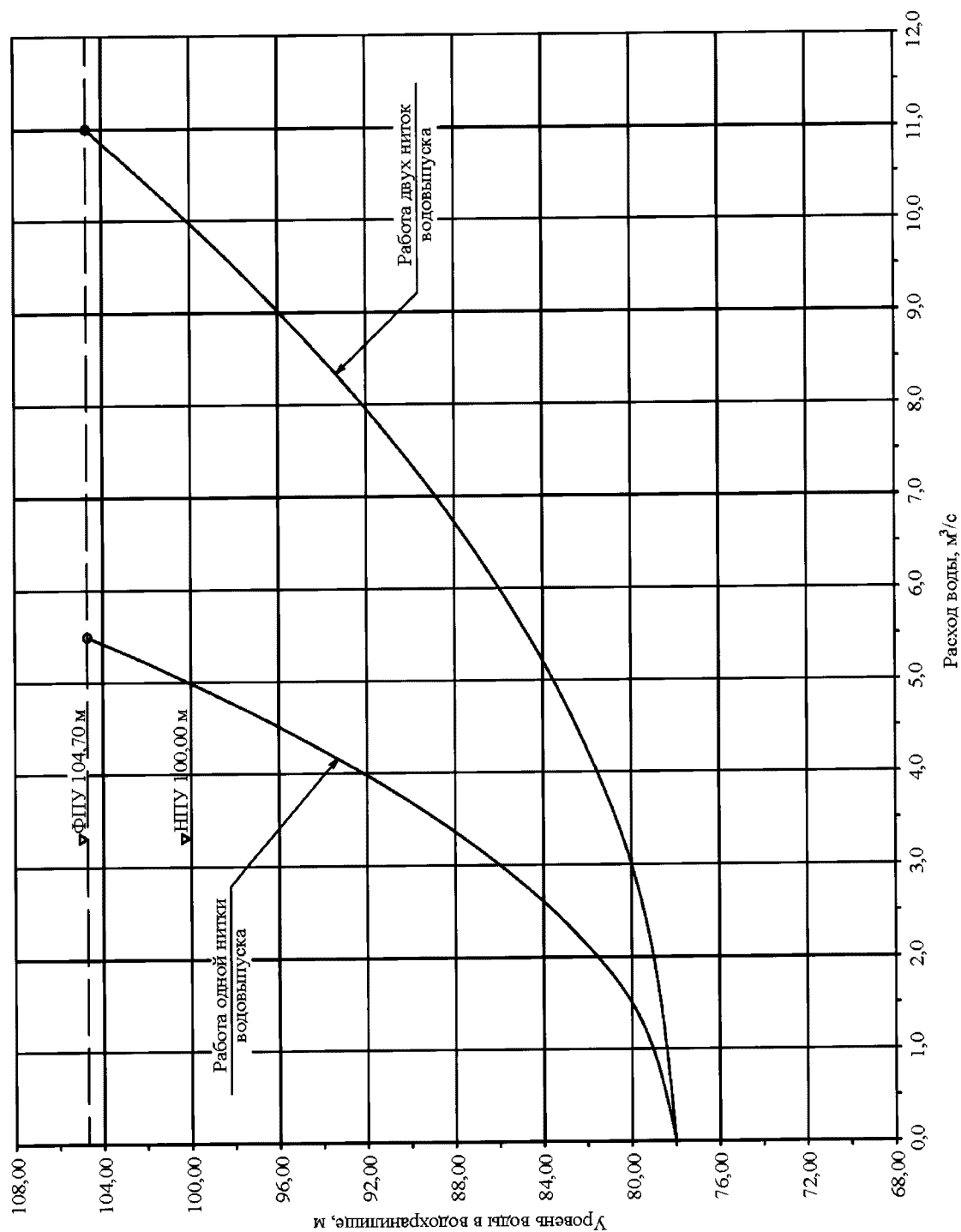
Пропускная способность донного водовыпуска-водозабора гидроузла Раковского водохранилища
