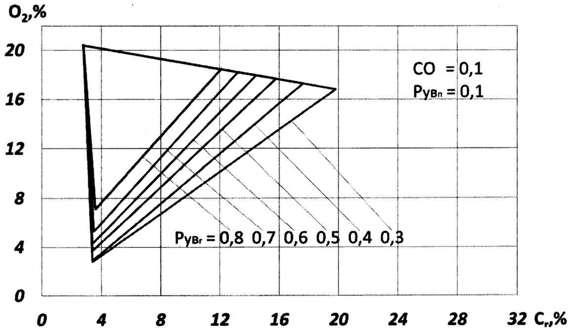
Рис. 14. Треугольник взрываемости при P_{CO} = 0,1 и P_{УВП} = 0,1
