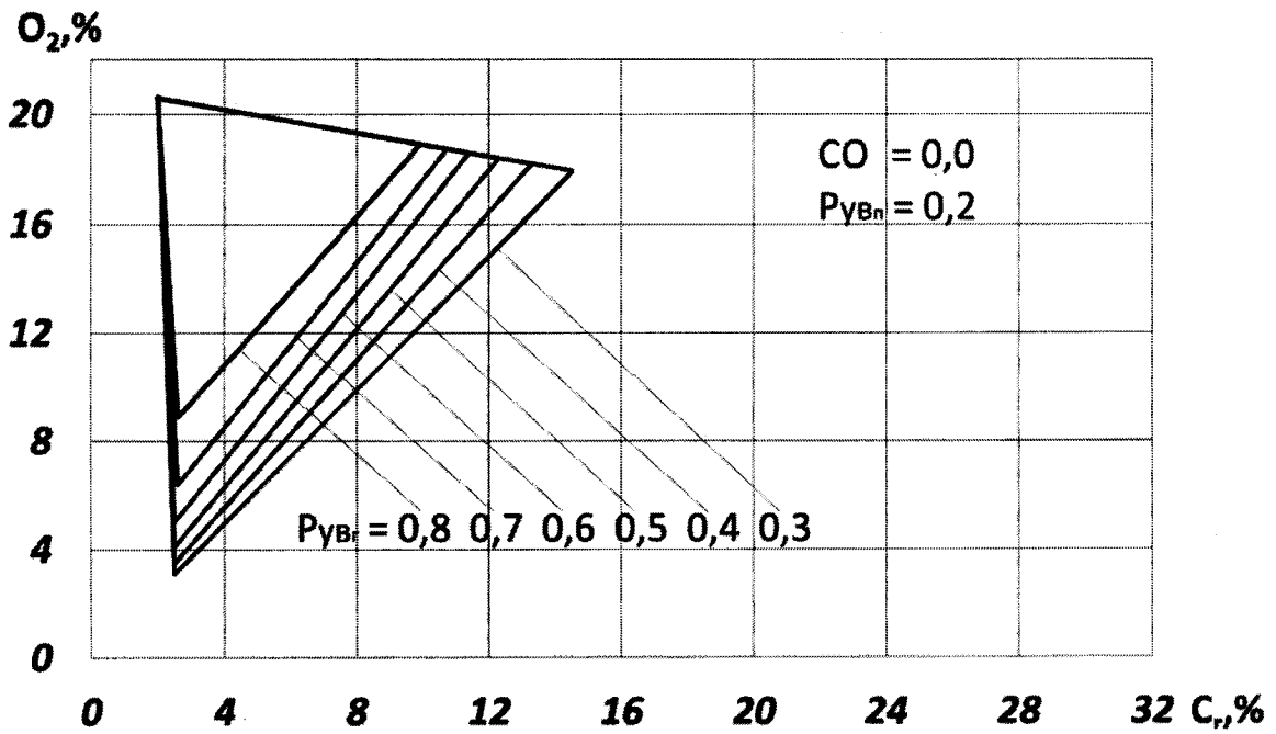
Рис. 12. Треугольник взрываемости при P_{CO} = 0,0 и P_{УВП} = 0,2
