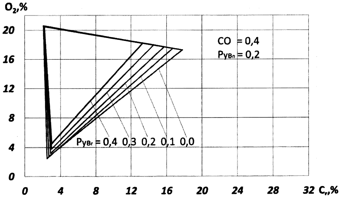
Рис. 24. Треугольник взрываемости при P_{CO} = 0,4 и P_{UВП} = 0,2
