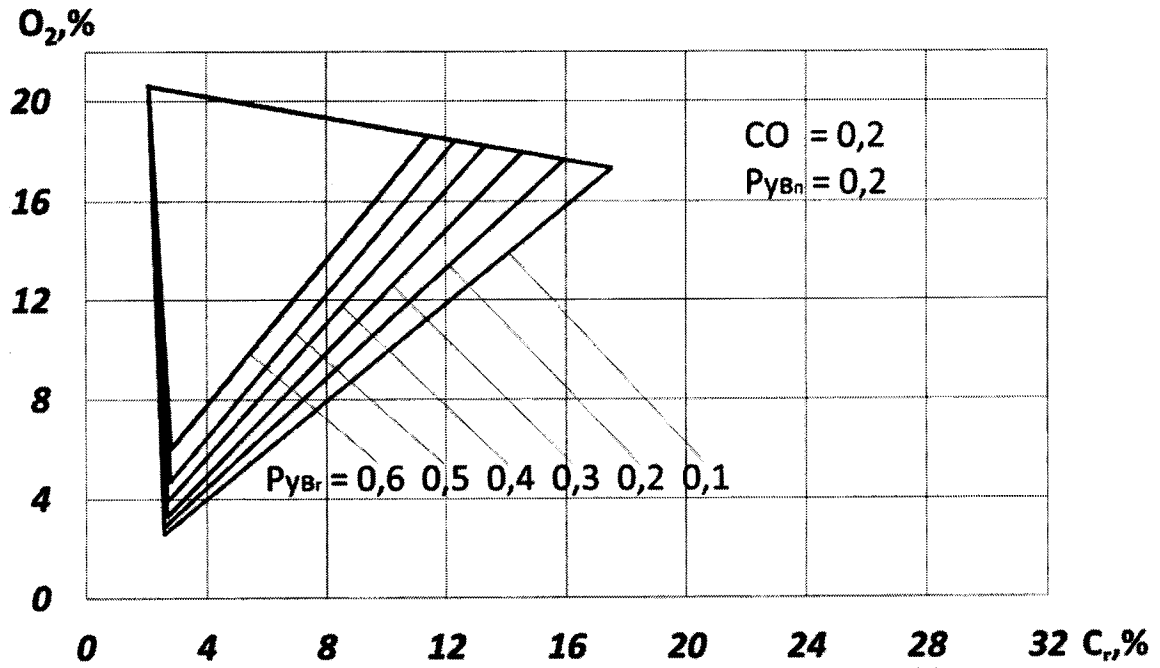
Рис. 18. Треугольник взрываемости при P_{CO} = 0,2 и P_{yBn} = 0,2
