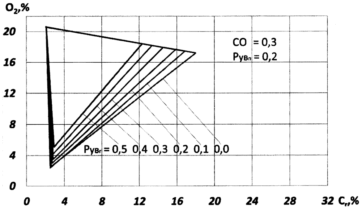
Рис. 21. Треугольник взрываемости при P_{CO} = 0,3 и P_{УВП} = 0,2
