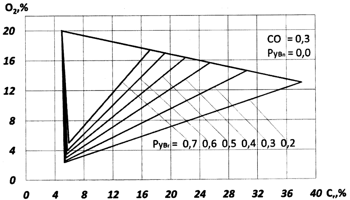
Рис. 19. Треугольник взрываемости при P_{CO} = 0,3 и P_{yBn} = 0,0
