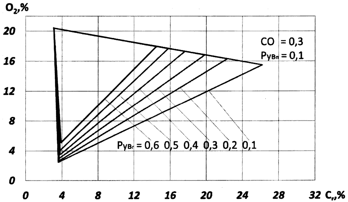
Рис. 20. Треугольник взрываемости при P_{CO} = 0,3 и P_{УВП} = 0,1
