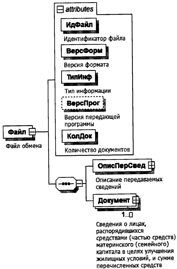
Рис.1. Диаграмма структуры файла обмена
