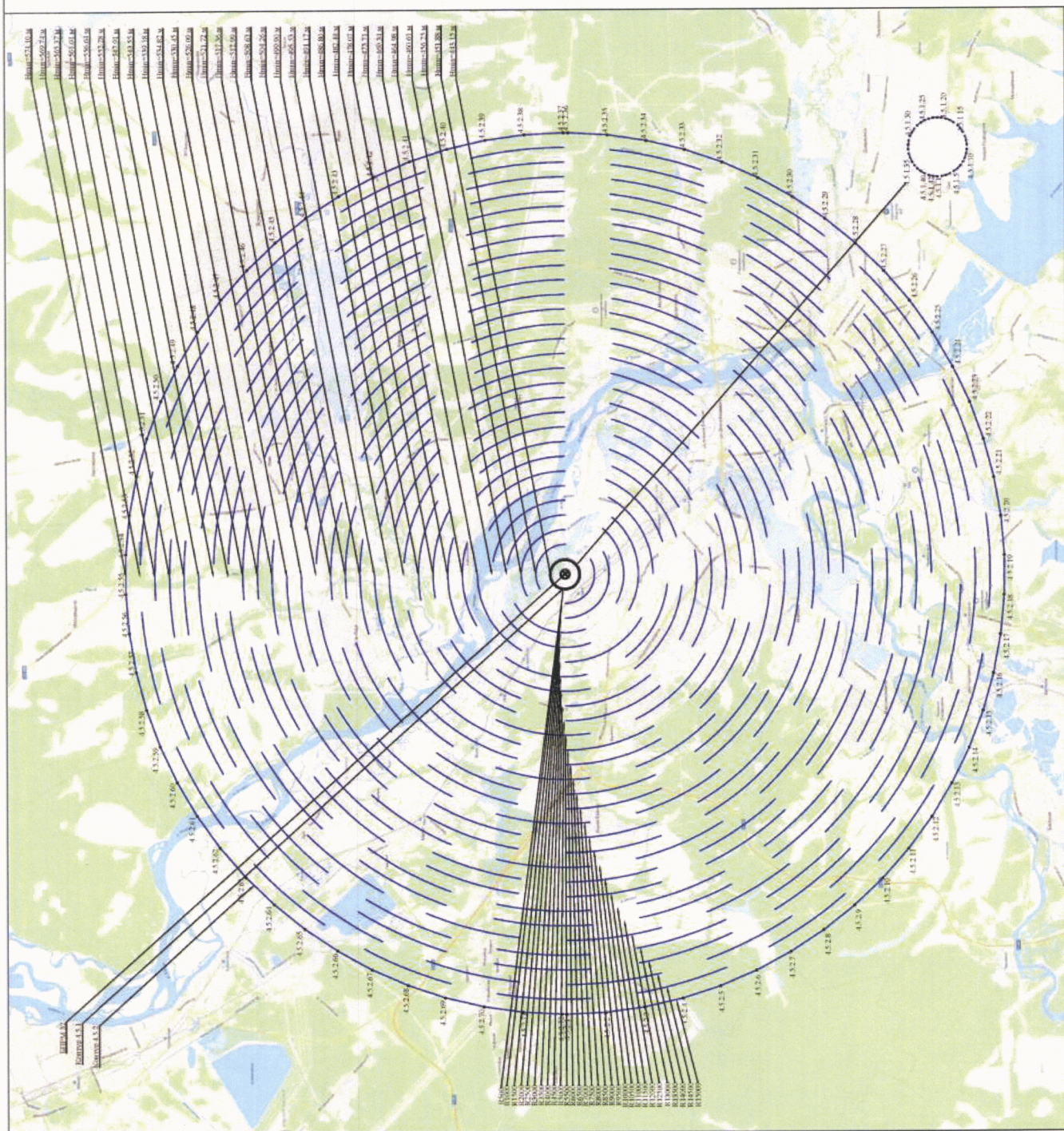
Схема 8.5 – зоны ограничения от ВРЛ-235 четвертой подзоны приаэродромной территории аэродрома Иркутск-2 (Восточный)
