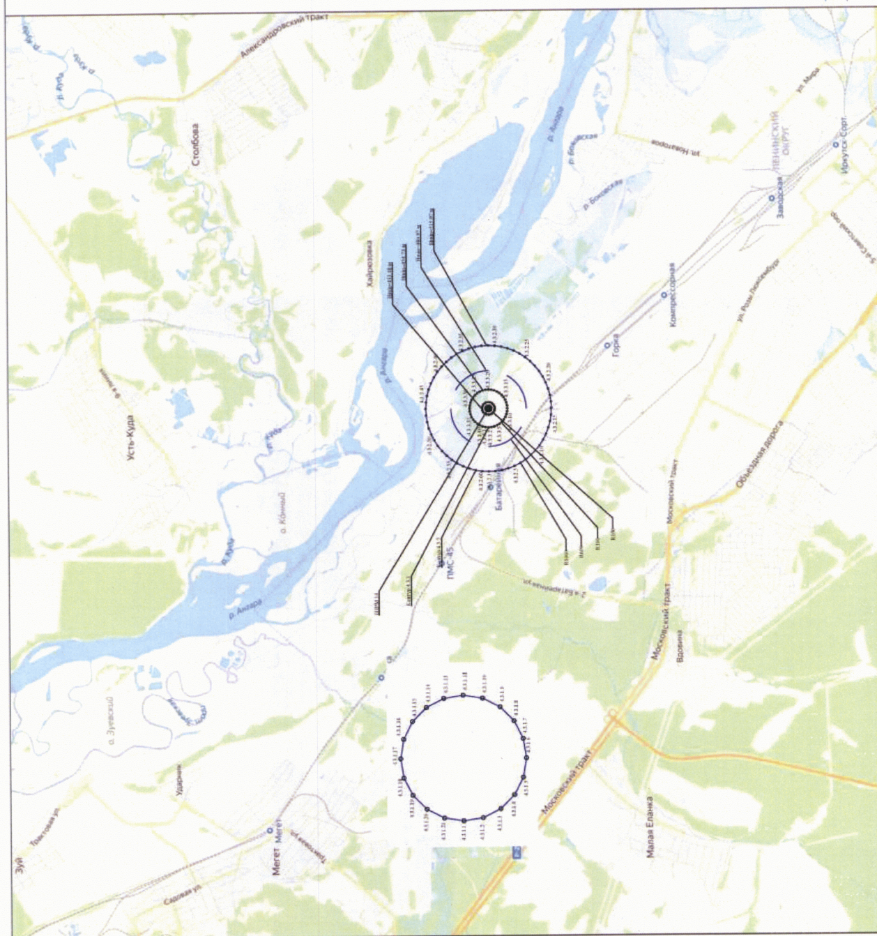
Схема 8.3 – зоны ограничения от БПРМ-14 четвертой подзоны приаэродромной территории аэродрома Иркутск-2 (Восточный)
