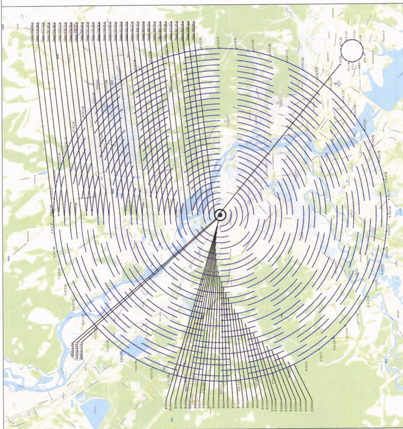
Схема 8.14 – зоны ограничения от ОРЛ-А-310 четвертой подзоны приаэродромной территории аэродрома Иркутск-2 (Восточный)
