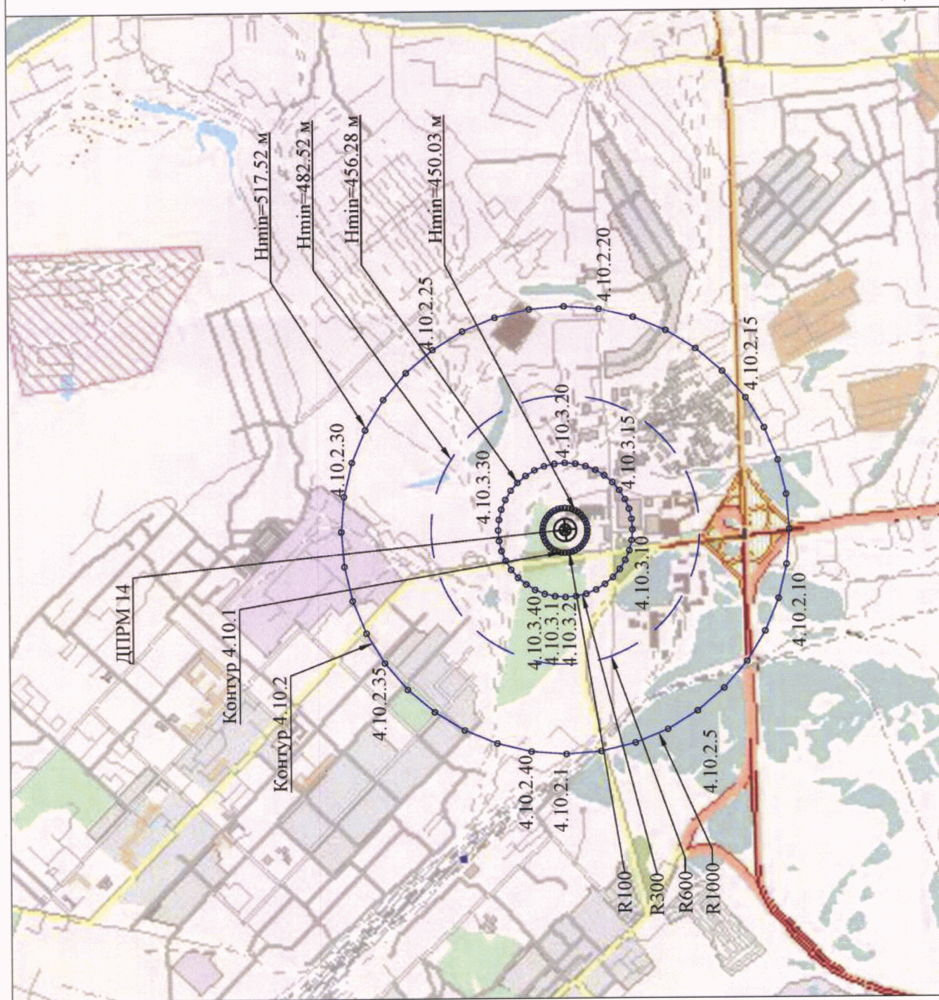
Схема 8.10 – зоны ограничения от ДПРМ-32 четвертой подзоны приаэродромной территории аэродрома Иркутск-2 (Восточный)
