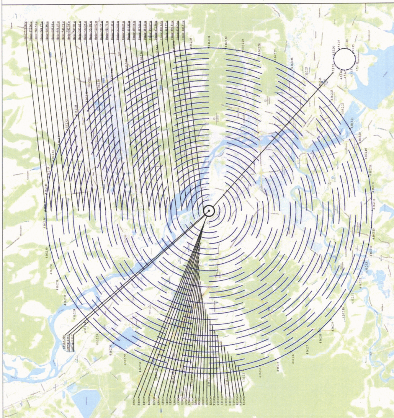
Схема 8.16 – зоны ограничения от ОРЛ-А-316 четвертой подзоны приаэродромной территории аэродрома Иркутск-2 (Восточный)
