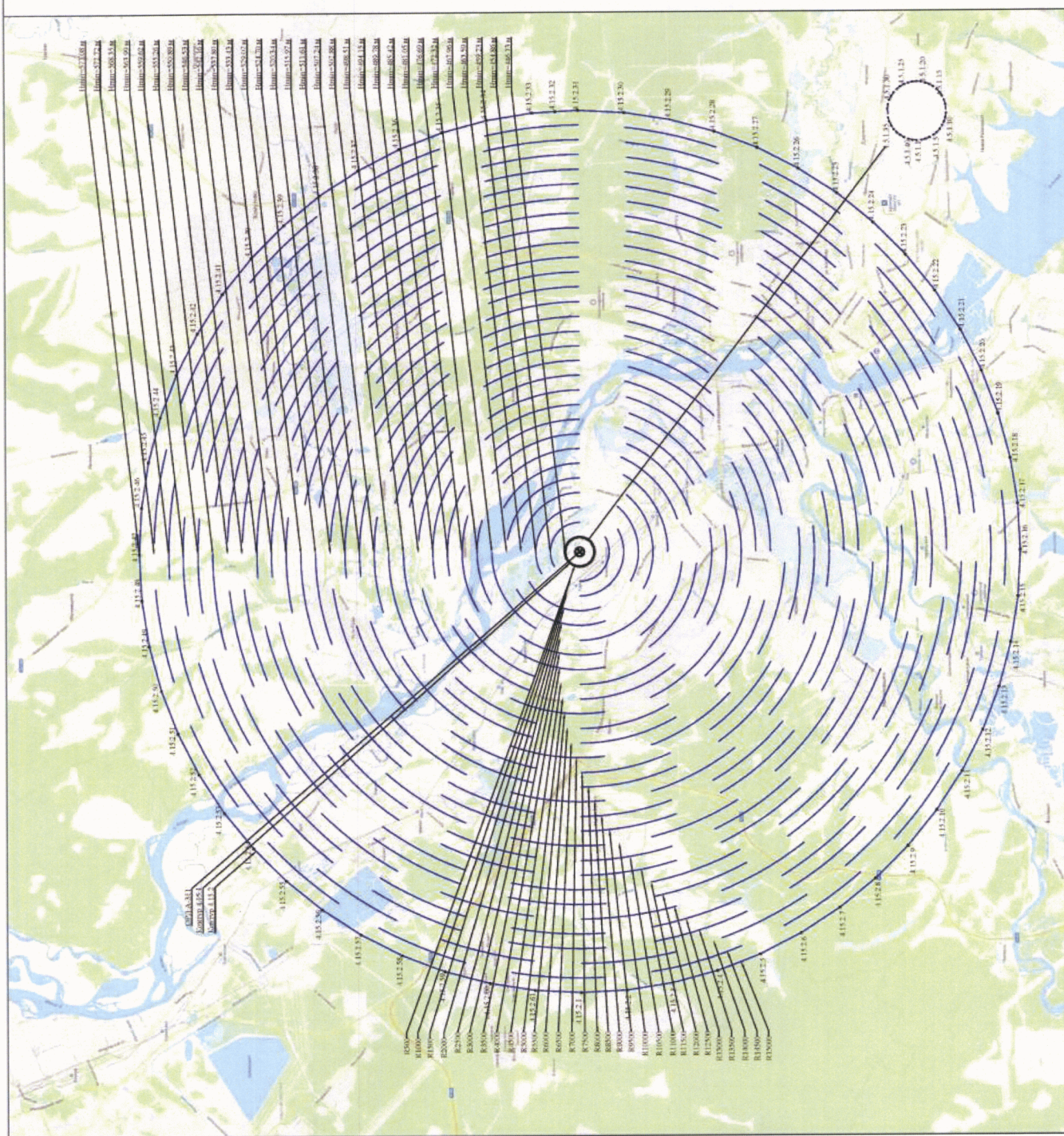
Схема 8.15 — зоны ограничения от ОРЛ-А-311 четвертой подзоны приаэродромной территории аэродрома Иркутск-2 (Восточный)
