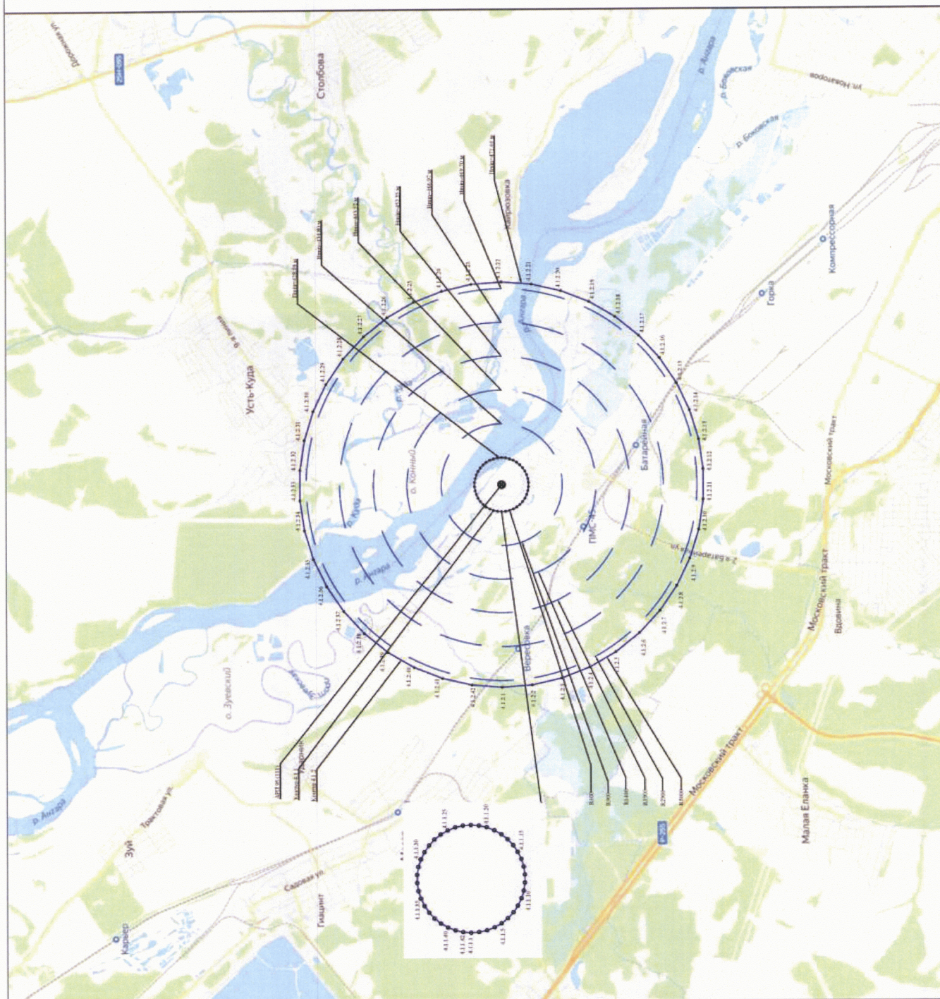
Схема 8.1 – зоны ограничения от АРП-95-111 четвертой подзоны приаэродромной территории аэродрома Иркутск-2 (Восточный)
