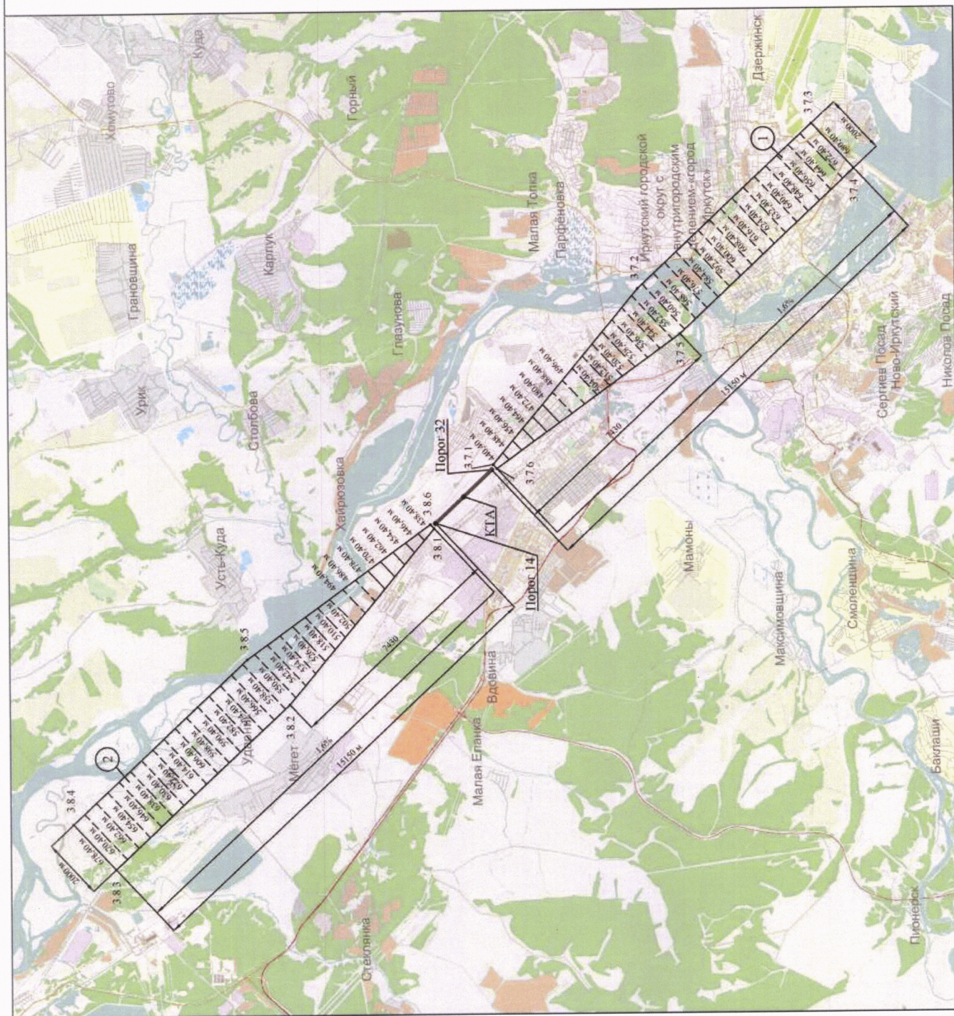
Схема 6.5 – ограничения препятствий для поверхностей взлета третьей подзоны приаэродромной территории аэродрома Иркутск-2 (Восточный)
