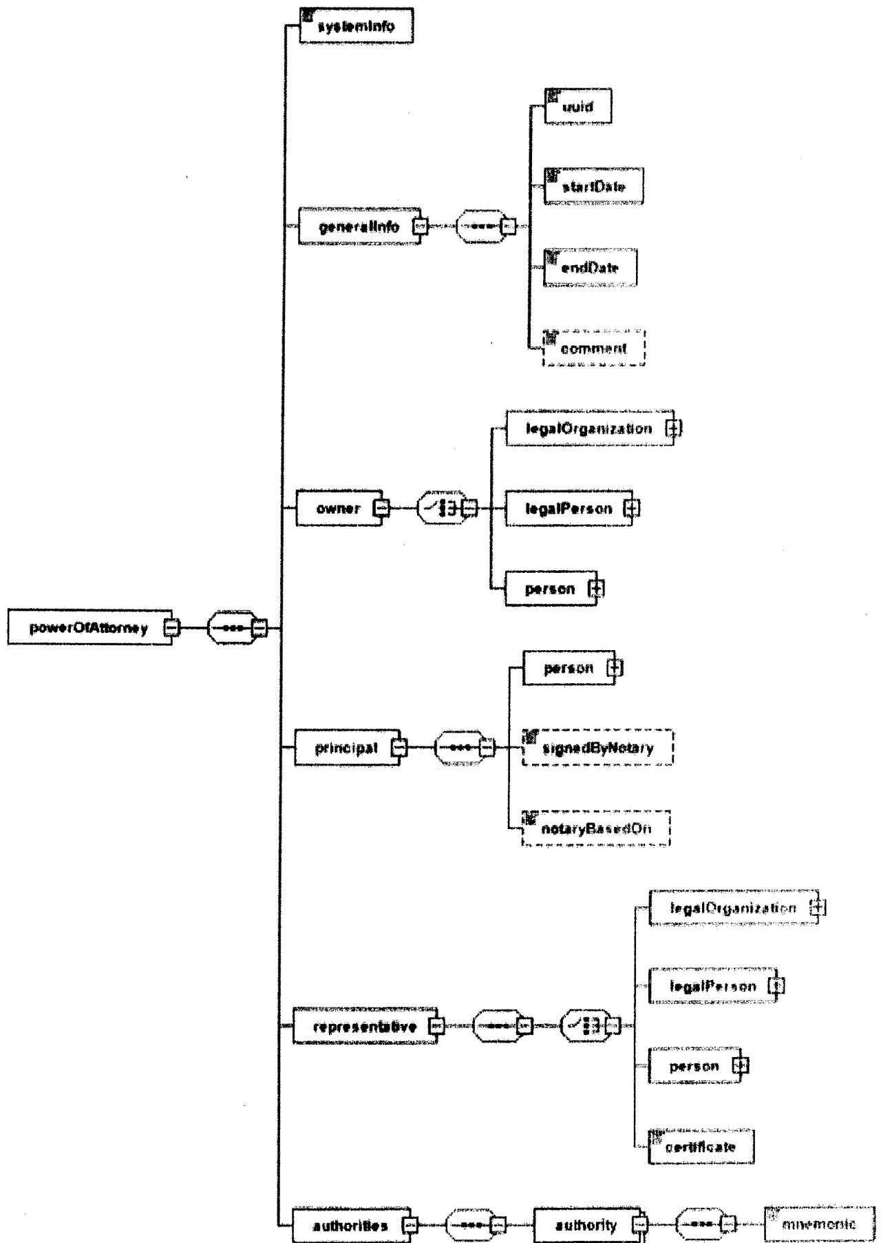
Рисунок. Диаграмма структуры файла обмена
