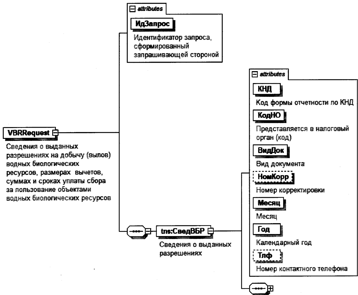
Рисунок 1. Диаграмма структуры документа обмена
