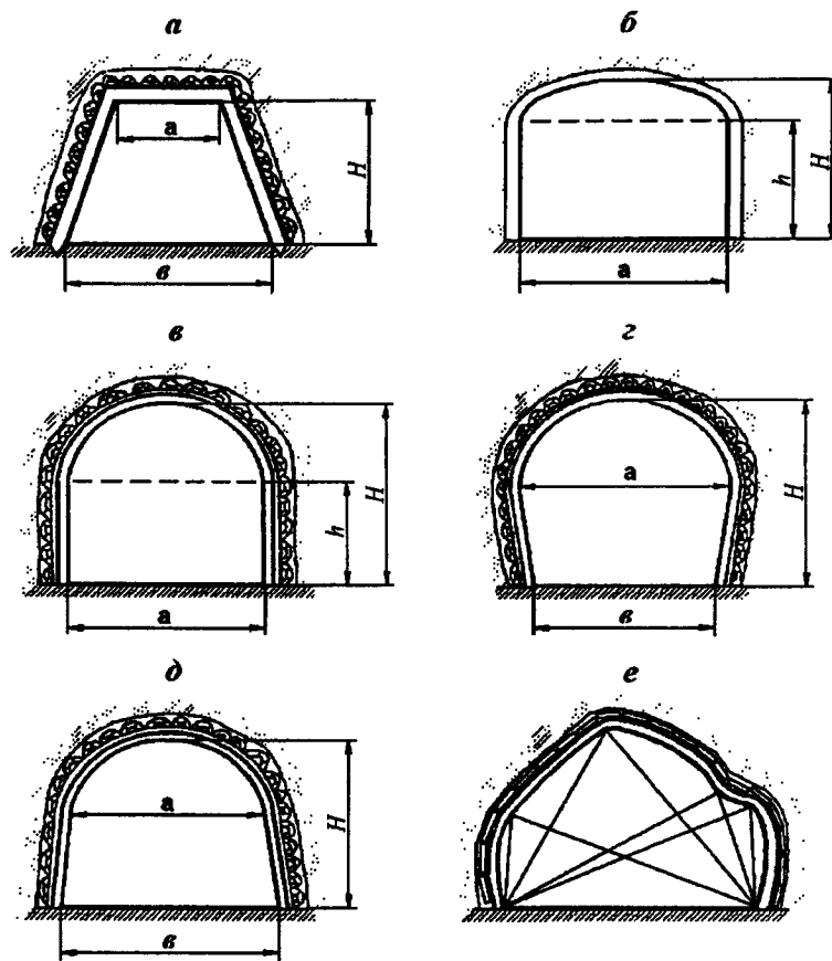
Рис. 2. Определение площадей поперечного сечения горных выработок:
