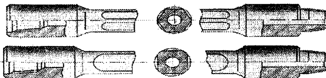
Рис. 121.2. Внешний вид ведущих бурильных труб
