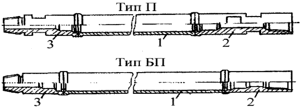
Рис. 121.3. Внешний вид бурильных труб
