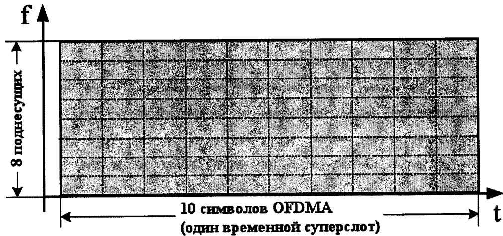
Рисунок 6. Структура подканала для временного суперслота
