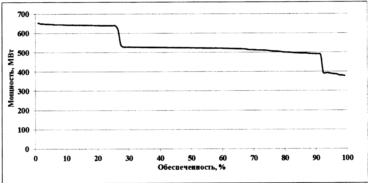
Вероятность превышения среднедекадных мощностей Зейской ГЭС за период с 1901/02 по 2016/17 гг. (первая декада июня)
