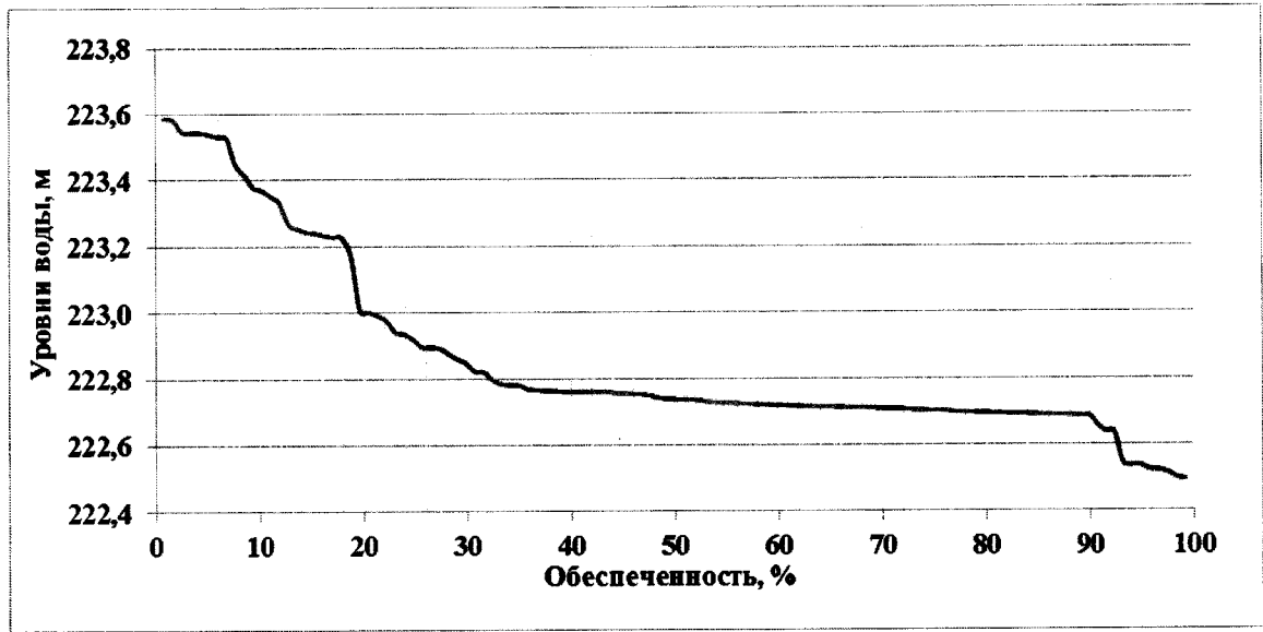
Вероятность превышения уровней нижнего бьефа Зейского гидроузла за период с 1901/02 по 2016/17 гг. (февраль)
