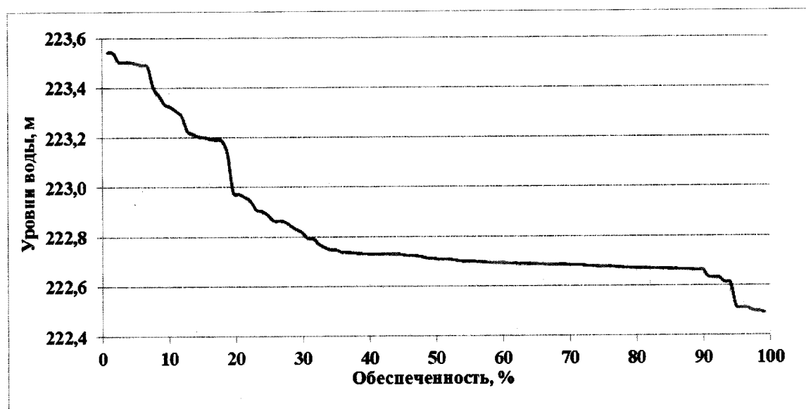
Вероятность превышения уровней нижнего бьефа Зейского гидроузла за период с 1901/02 по 2016/17 гг. (декабрь)
