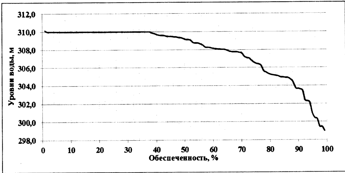
Вероятность превышения уровней воды Зейского водохранилища на конец интервала за период с 1901/02 по 2016/17 гг. (апрель)
