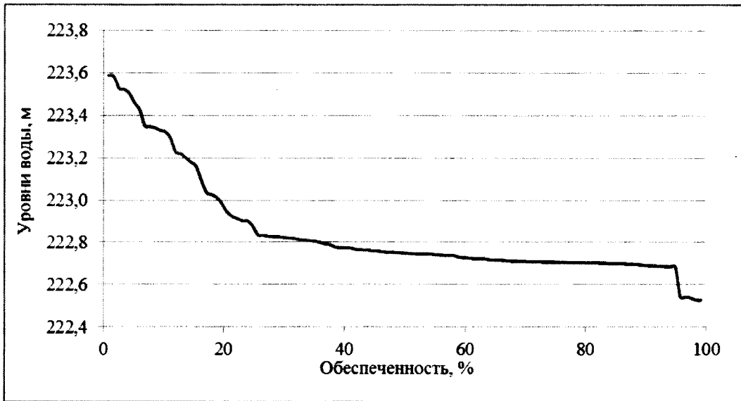
Вероятность превышения уровней нижнего бьефа Зейского гидроузла за период с 1901/02 по 2016/17 гг. (февраль)
