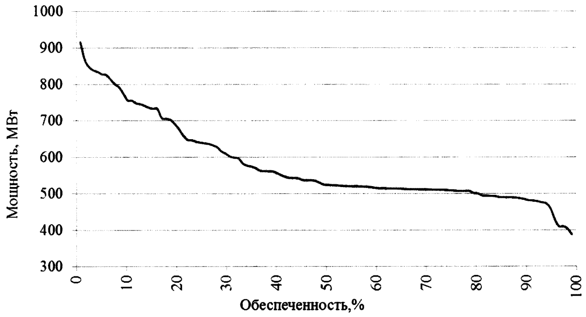
Вероятность превышения среднегодовых мощностей Зейской ГЭС за период с 1901/02 по 2016/17 гг.
