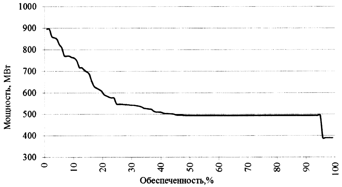
Вероятность превышения среднемесячных мощностей Зейской ГЭС за период с 1901/02 по 2016/17 гг. (март)
