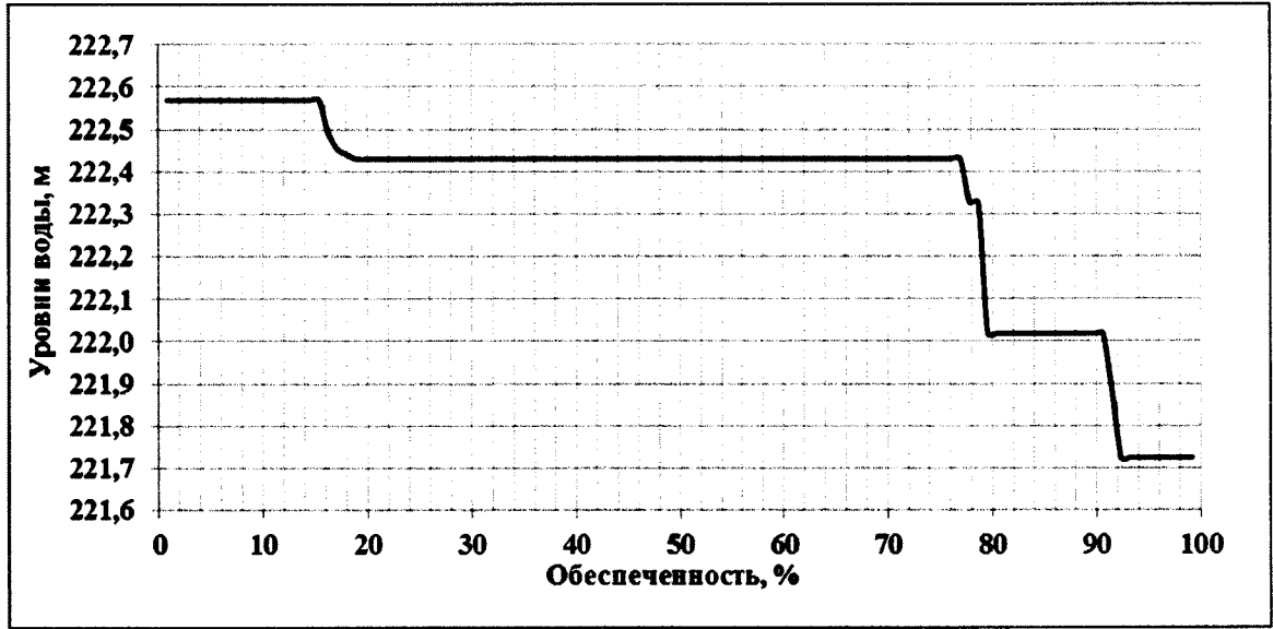
Вероятность превышения уровней нижнего бьефа Зейского гидроузла за период с 1901/02 по 2016/17 гг. (вторая - третья декада июня)
