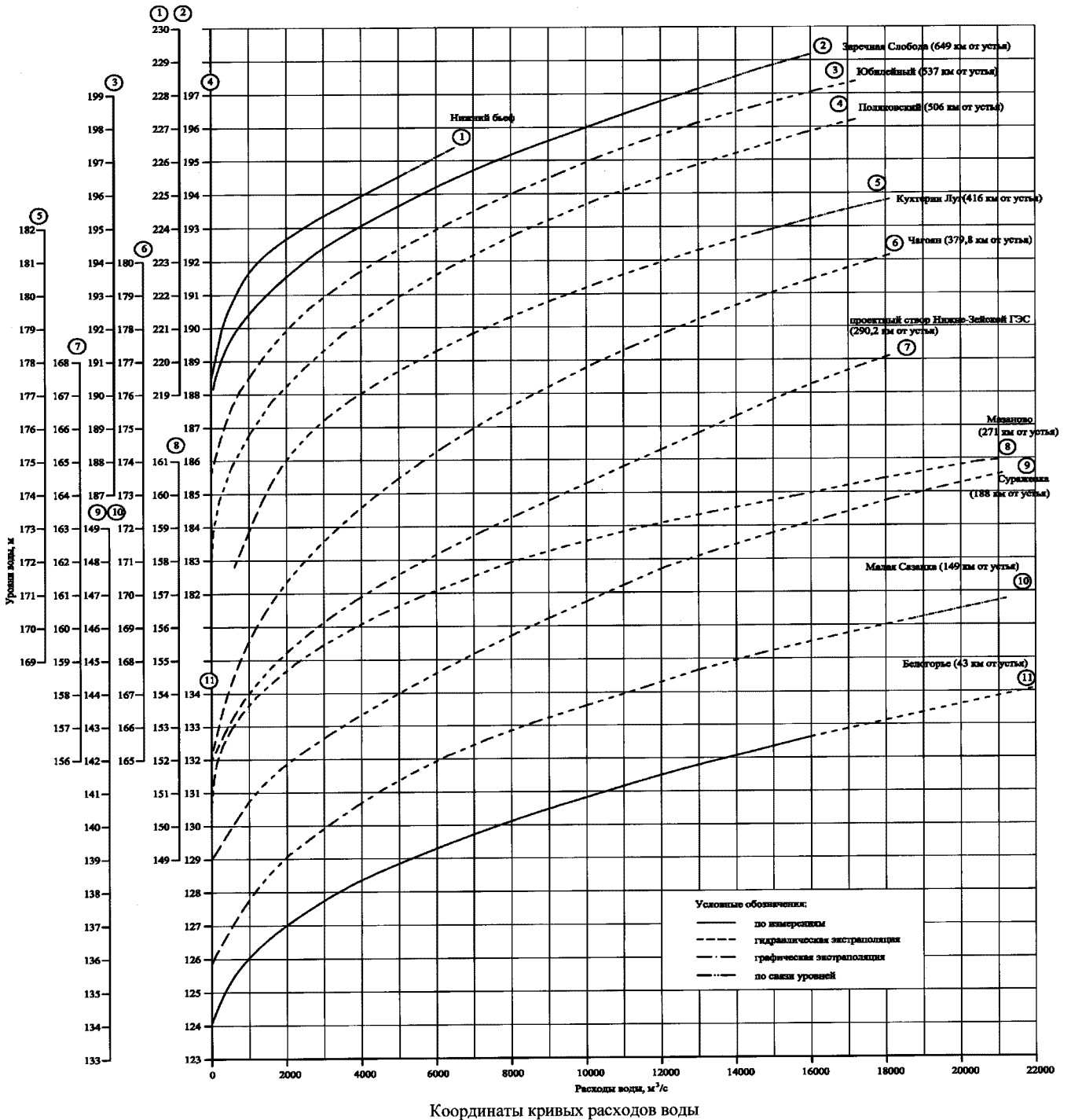
Координаты кривых расходов воды
