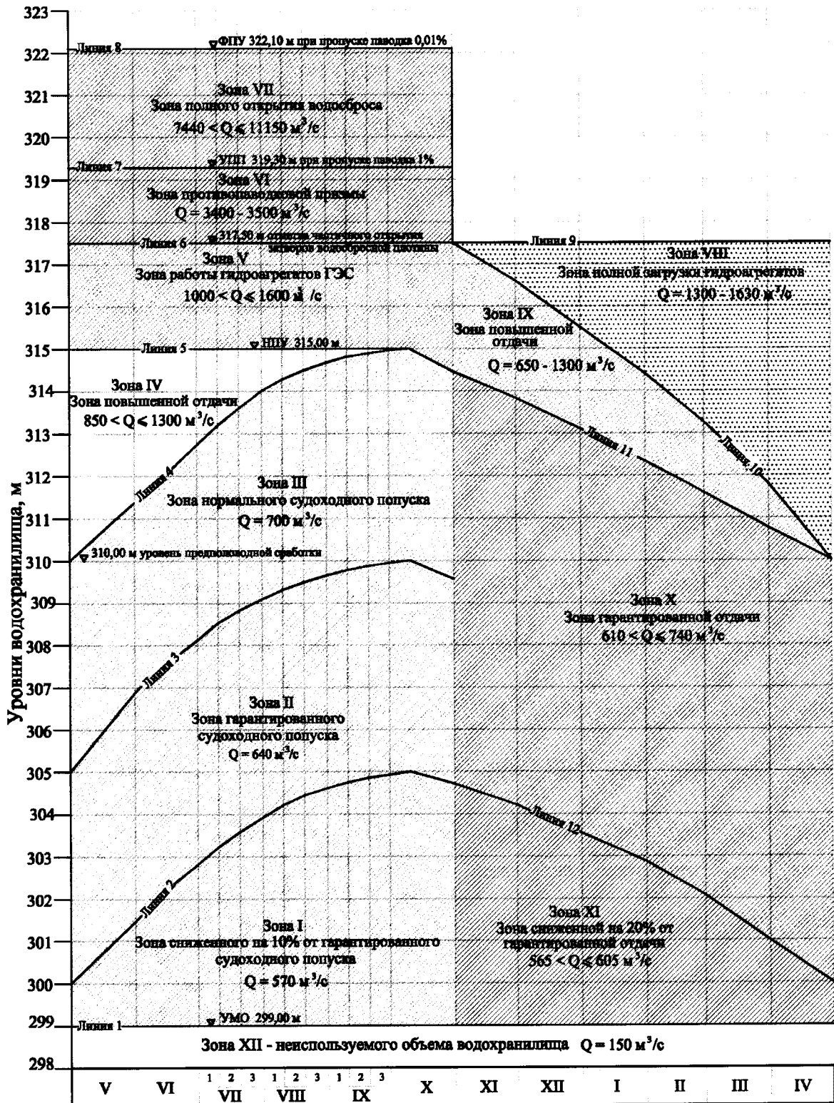
Диспетчерский график работы Зейского водохранилища
