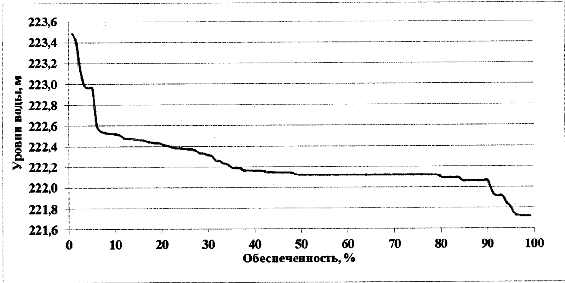
Вероятность превышения уровней нижнего бьефа Зейского гидроузла за период с 1901/02 по 2016/17 гг. (летний период)
