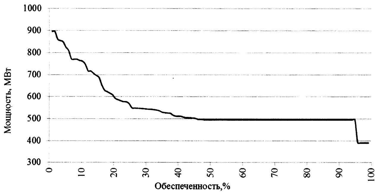
Вероятность превышения среднемесячных мощностей Зейской ГЭС за период с 1901/02 по 2016/17 гг. (декабрь)
