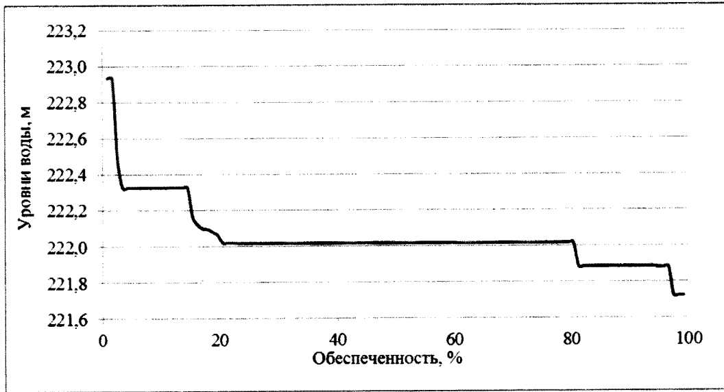
Вероятность превышения уровней нижнего бьефа Зейского гидроузла за период с 1901/02 по 2016/17 гг. (июнь)
