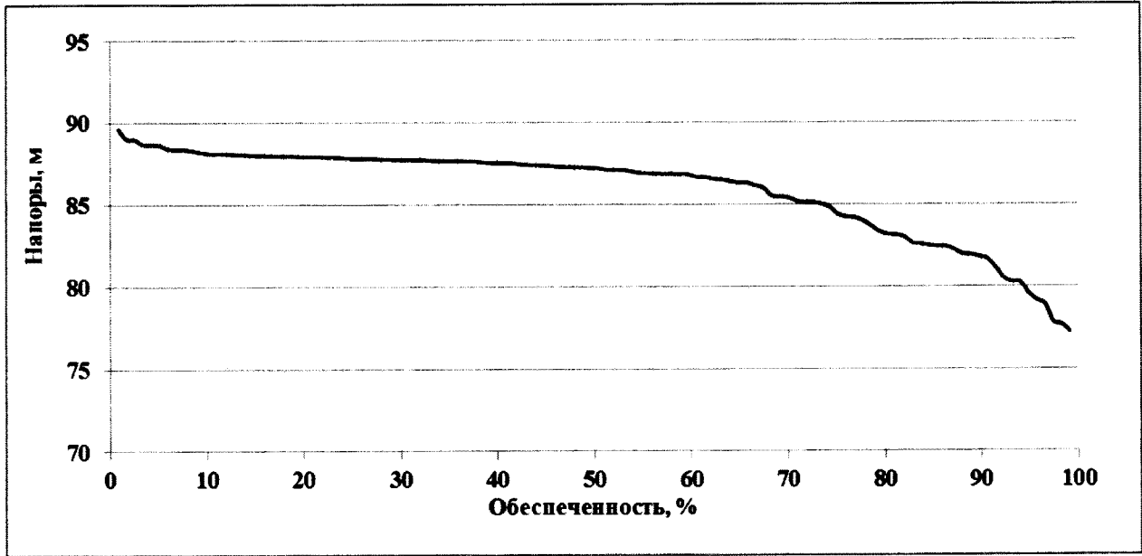
Вероятность превышения среднедекадных напоров-нетто на Зейском гидроузле за период с 1901/02 по 2016/17 гг. (первая декада июня)
