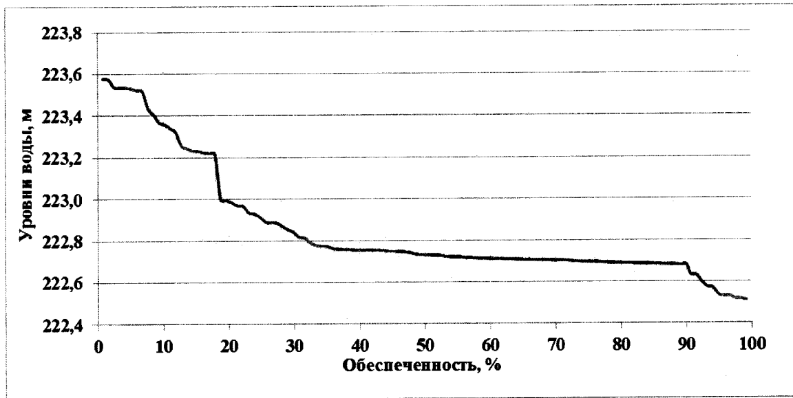
Вероятность превышения уровней нижнего бьефа Зейского гидроузла за период с 1901/02 по 2016/17 гг. (зимний период)
