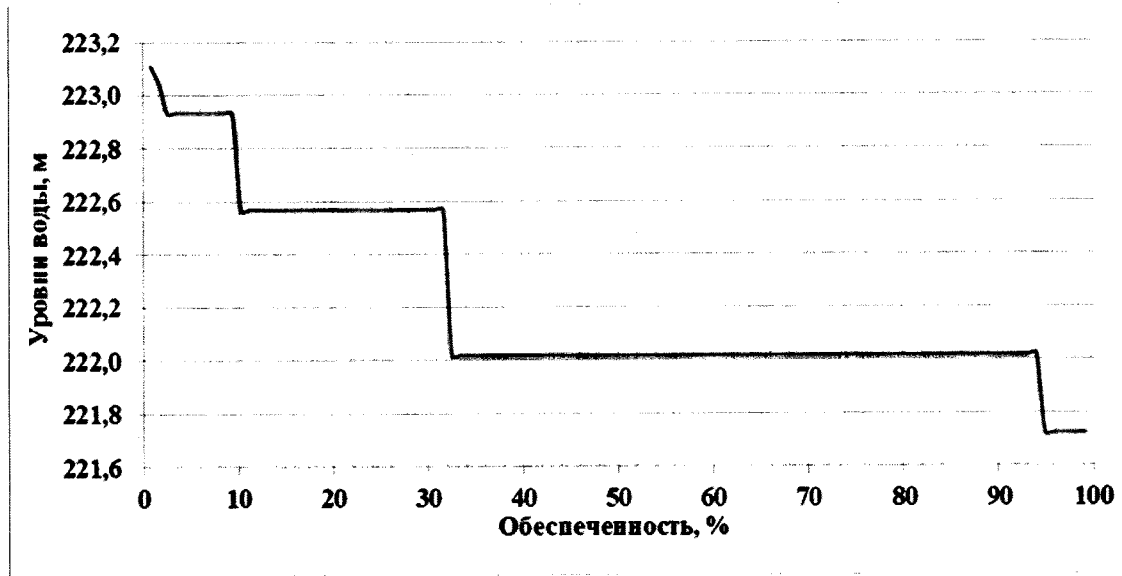
Вероятность превышения уровней нижнего бьефа Зейского гидроузла за период с 1901/02 по 2016/17 гг. (первая декада октября)
