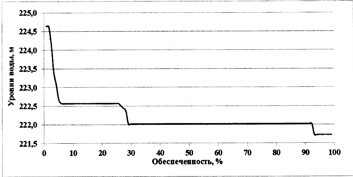
Вероятность превышения уровней нижнего бьефа Зейского гидроузла за период с 1901/02 по 2016/17 гг. (третья декада августа)
