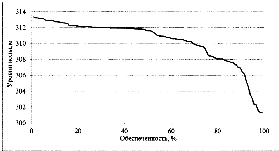
Вероятность превышения уровней воды Зейского водохранилища на конец интервала за период с 1901/02 по 2016/17 гг. (зимний период)
