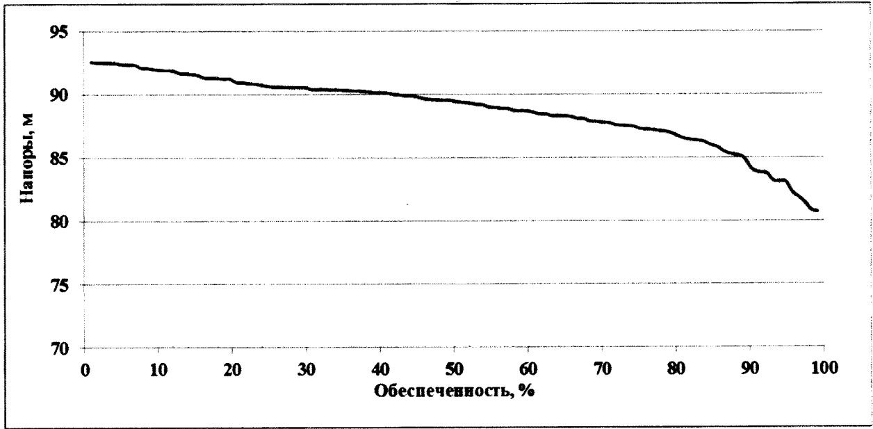
Вероятность превышения среднедекадных напоров-нетто на Зейском гидроузле за период с 1901/02 по 2016/17 гг. (первая декада сентября)
