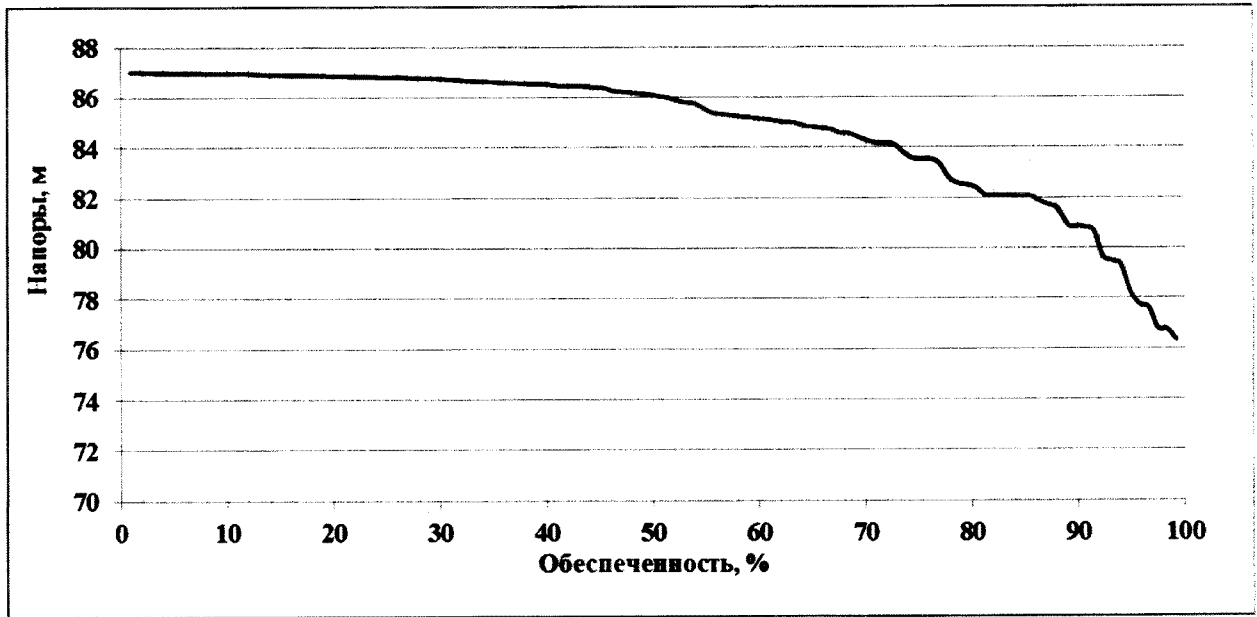
Вероятность превышения среднемесячных напоров-нетто на Зейском гидроузле за период с 1901/02 по 2016/17 гг. (март)
