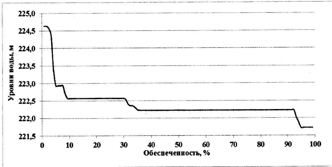
Вероятность превышения уровней нижнего бьефа Зейского гидроузла за период с 1901/02 по 2016/17 гг. (вторая декада сентября)
