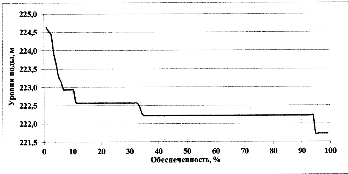
Вероятность превышения уровней нижнего бьефа Зейского гидроузла за период с 1901/02 по 2016/17 гг. (третья декада сентября)
