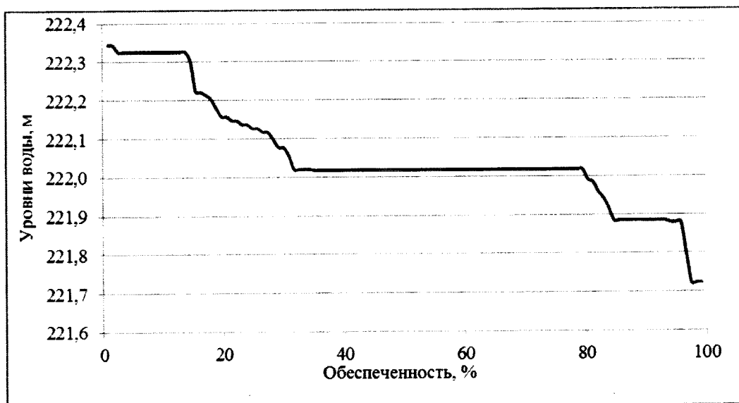
Вероятность превышения уровней нижнего бьефа Зейского гидроузла за период с 1901/02 по 2016/17 гг. (май)
