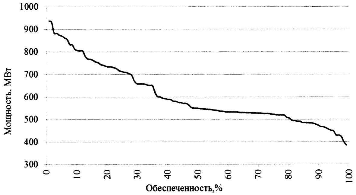
Вероятность превышения средних мощностей Зейской ГЭС за период с 1901/02 по 2016/17 гг. (летний период)
