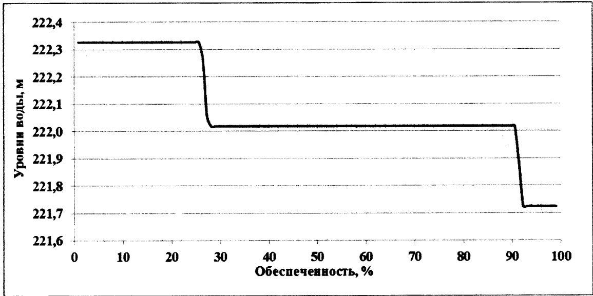
Вероятность превышения уровней нижнего бьефа Зейского гидроузла за период с 1901/02 по 2016/17 гг. (первая декада июня)
