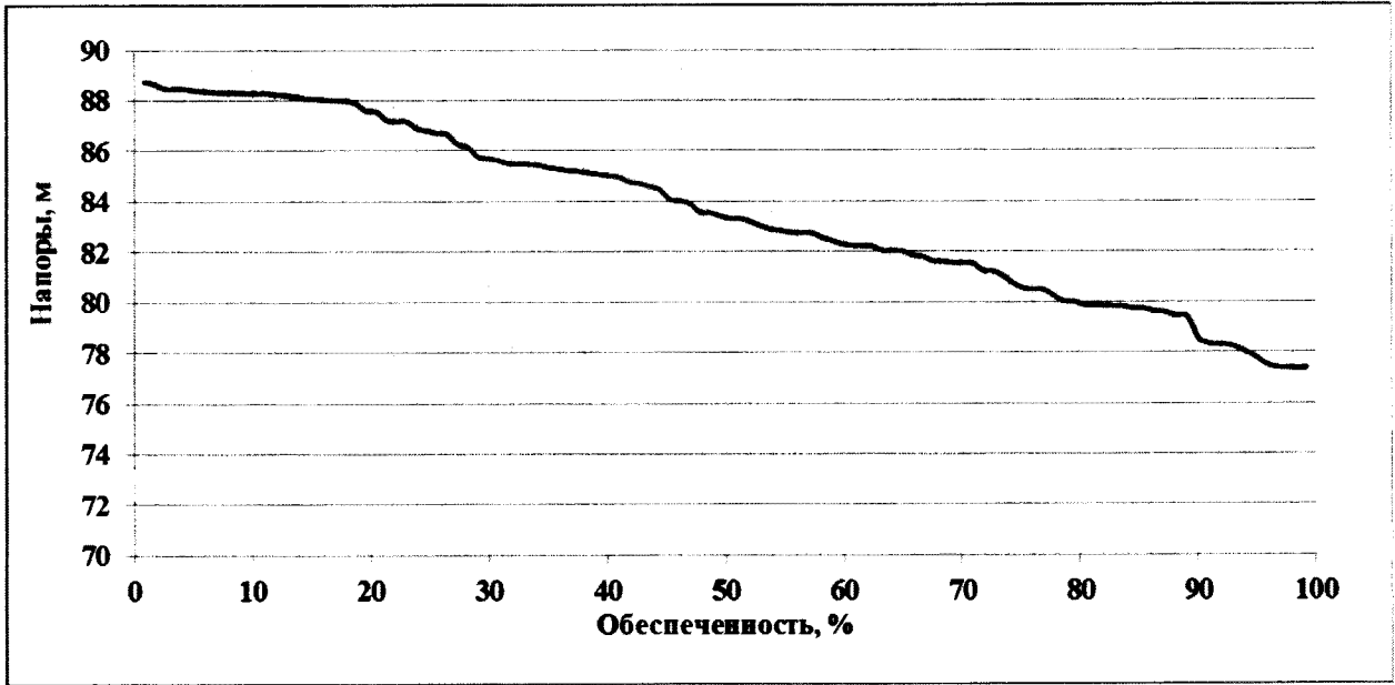
Вероятность превышения средних напоров-нетто на Зейском гидроузле за период с 1901/02 по 2016/17 гг. (зимний период)
