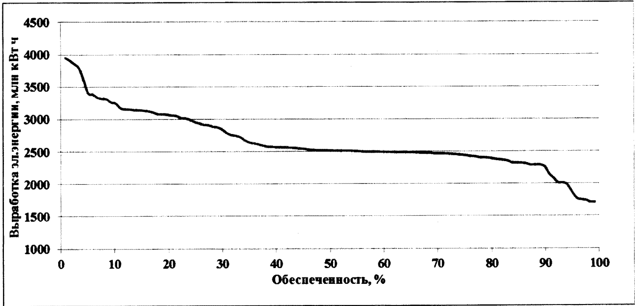
Вероятность превышения суммарного объема выработки электроэнергии Зейской ГЭС за период с 1901/02 по 2016/17 гг. (зимний период)
