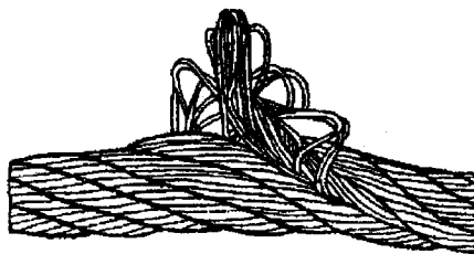
Рисунок 11. Выдавливание сердечника
