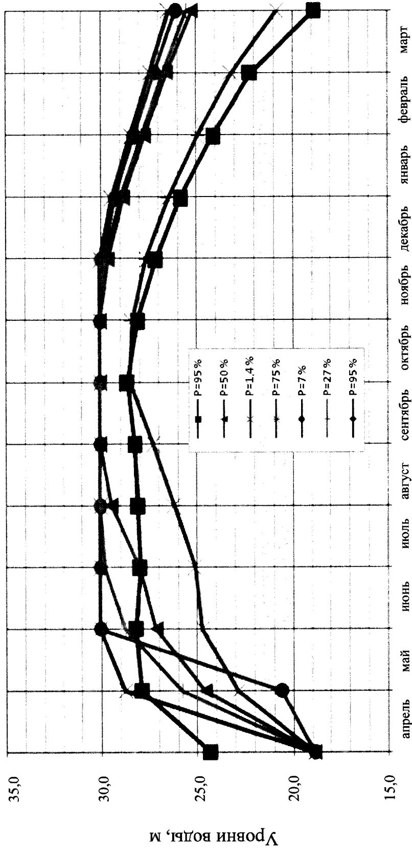
Кривые продолжительности конечных для интервалов регулирования уровней воды в верхнем бьефе гидроузла Пионерского водохранилища
