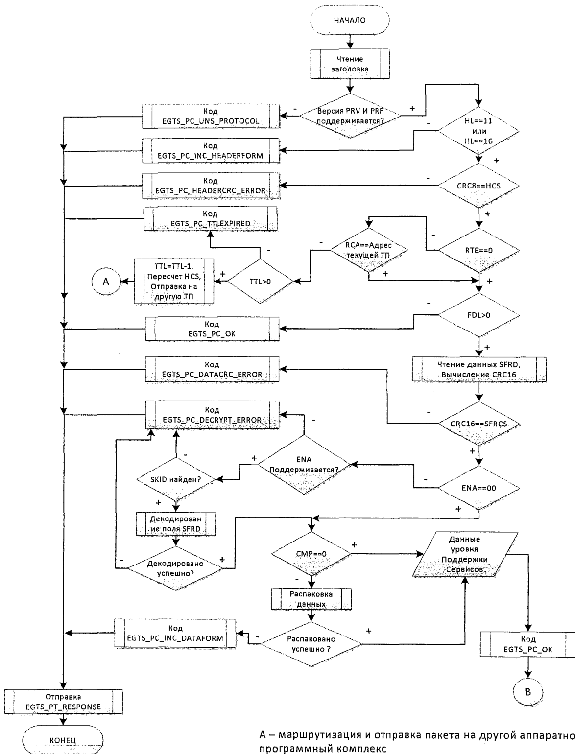
Рисунок 2. Блок-схема алгоритма обработки пакета данных протокола Транспортного уровня при приеме
