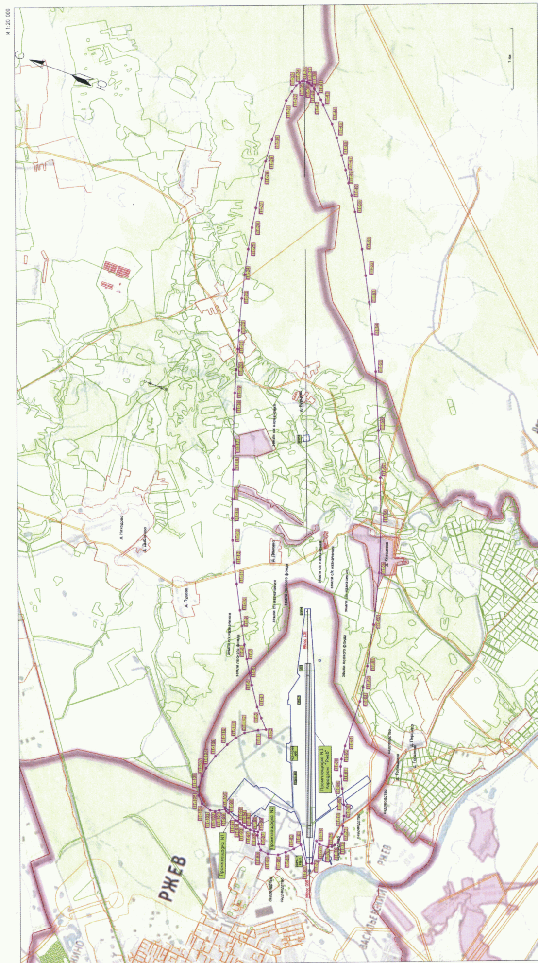
Схема № 11 - граница седьмой подзоны приаэродромной территории аэродрома экспериментальной авиации Ржев
