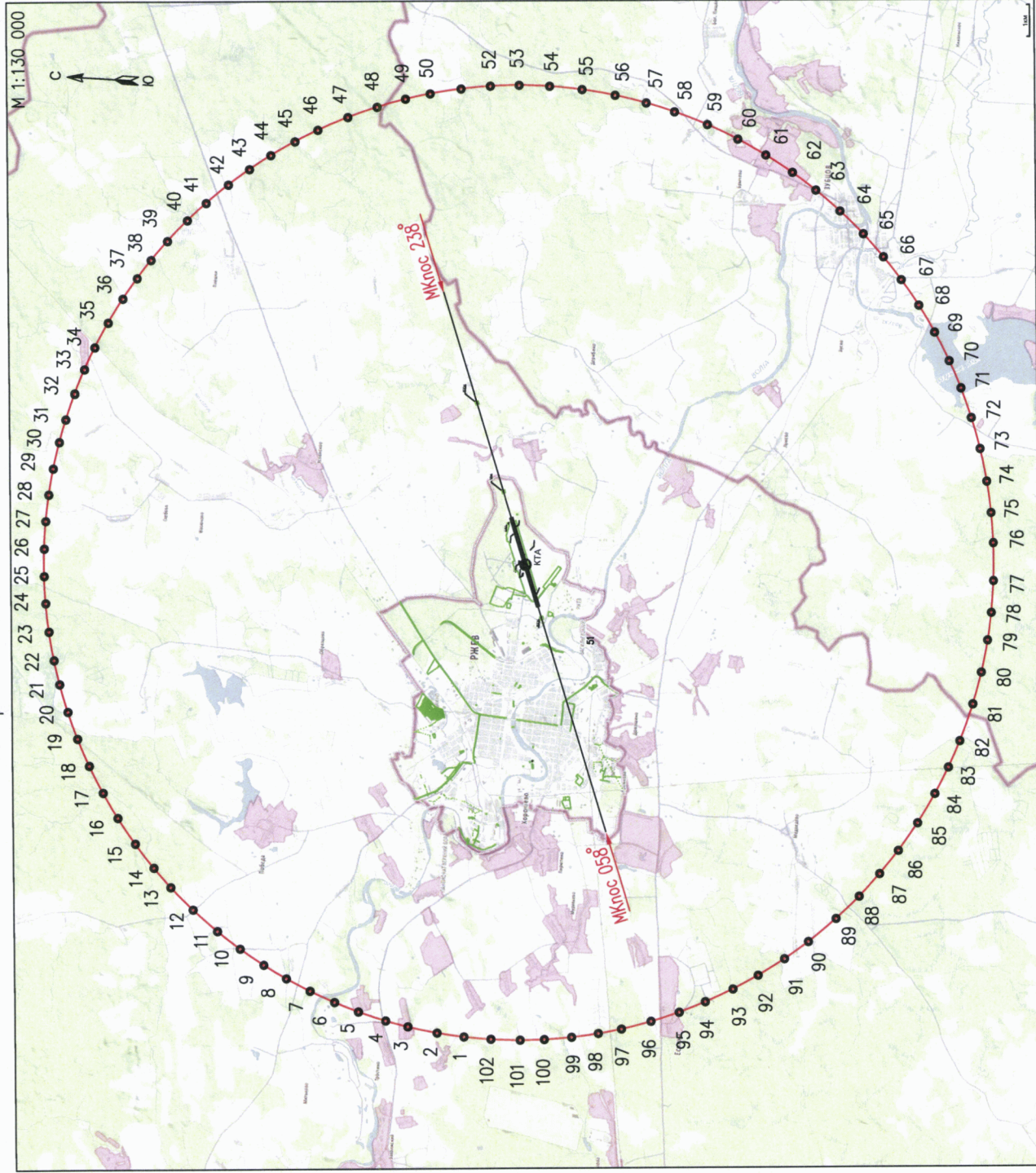
Схема № 6 - граница четвертой подзоны приаэродромной территории аэродрома экспериментальной авиации Ржев
