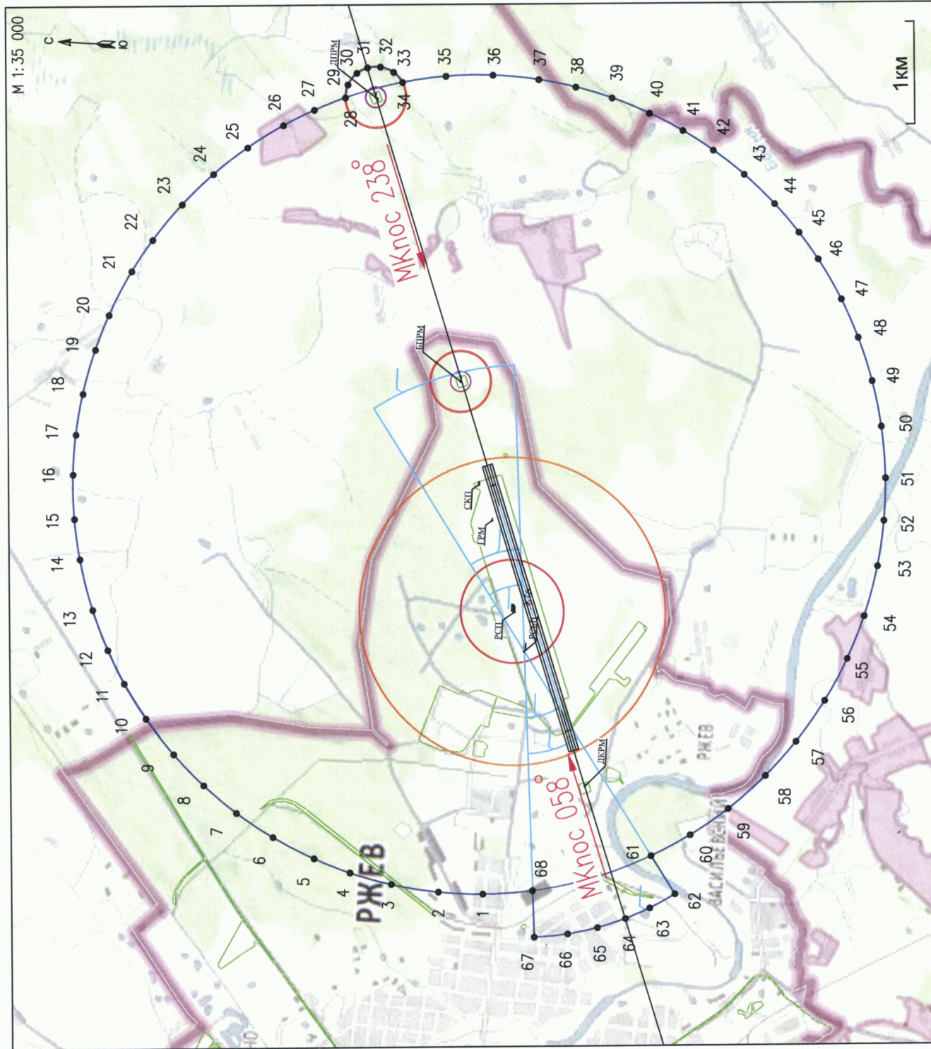
Схема № 7 - границы охранных зон от воздействия промышленных помех четвертой подзоны приаэродромной территории аэродрома экспериментальной авиации Ржев
