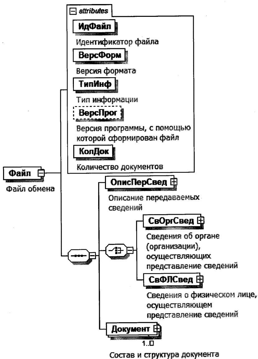
Рисунок 1. Диаграмма структуры файла обмена
