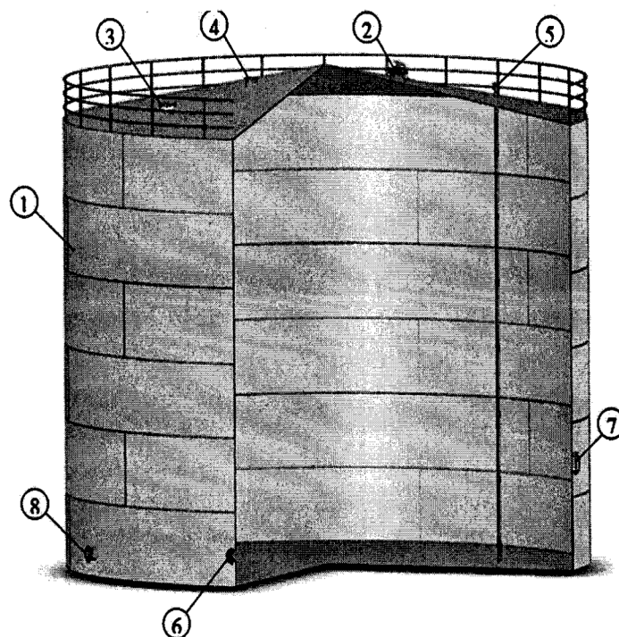
Рис. 117.2 Типовая схема вертикального цилиндрического стального резервуара
