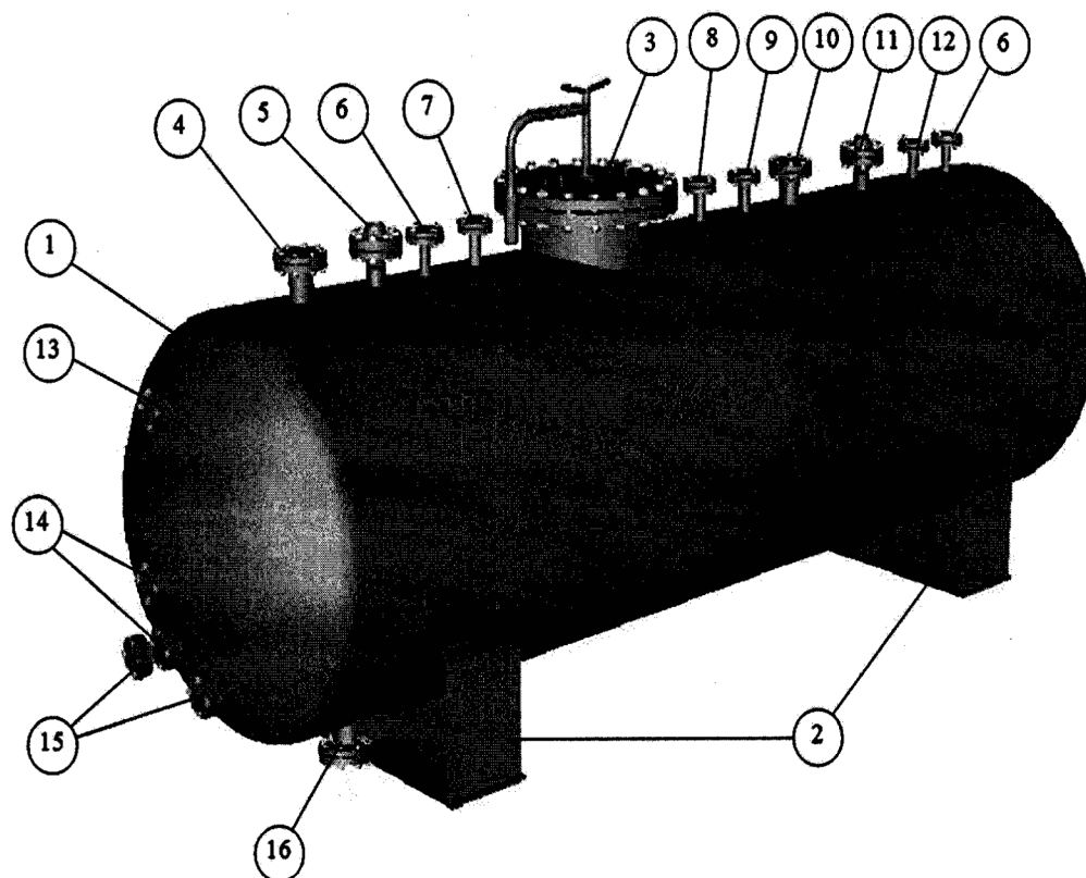
Рис. 117.3 Типовая емкость малой вместимости
