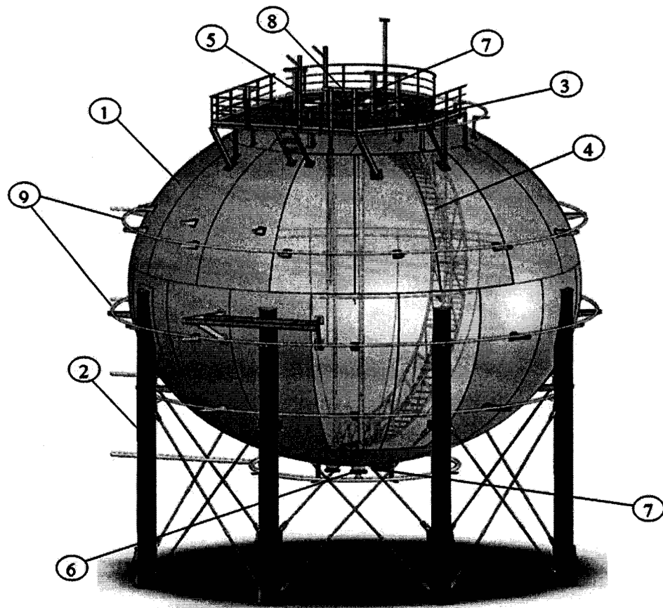
Рис. 120.2 Типовая схема шарового резервуара
