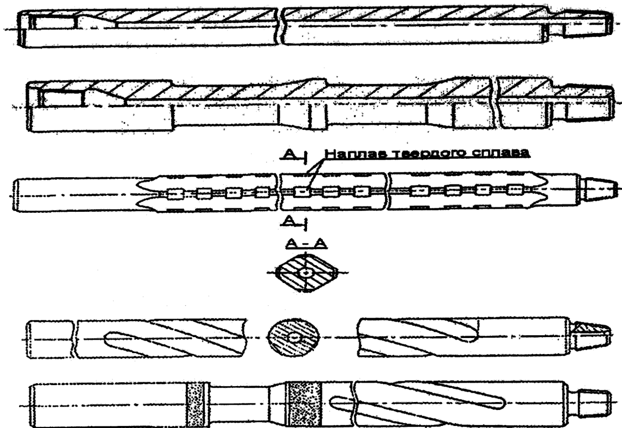
Рис. 133.1 Внешний вид утяжеленных бурильных труб
