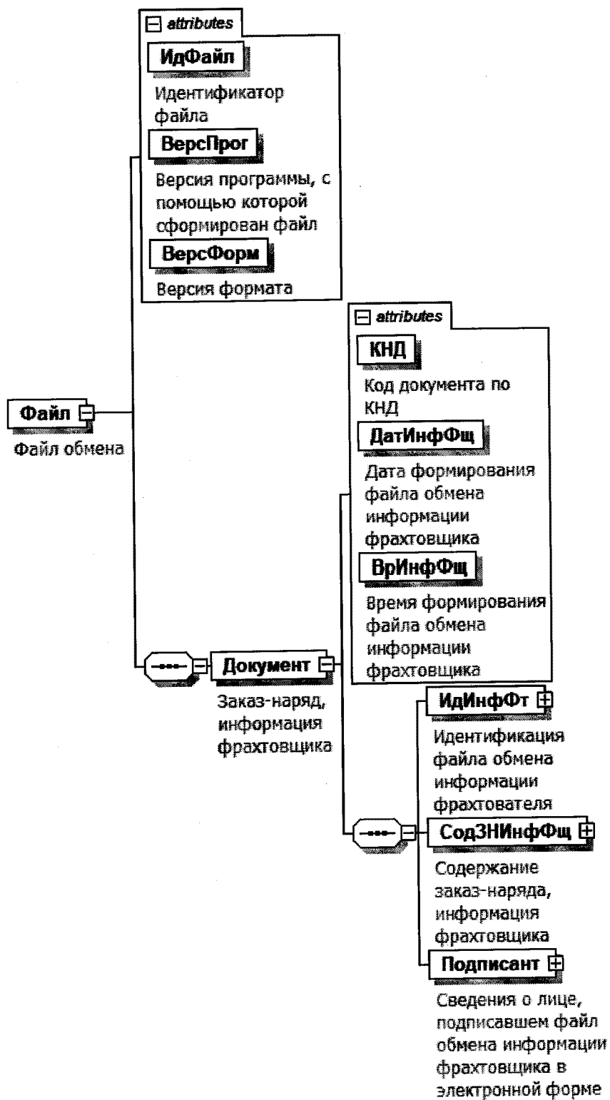
Рисунок 2. Диаграмма структуры файла обмена
