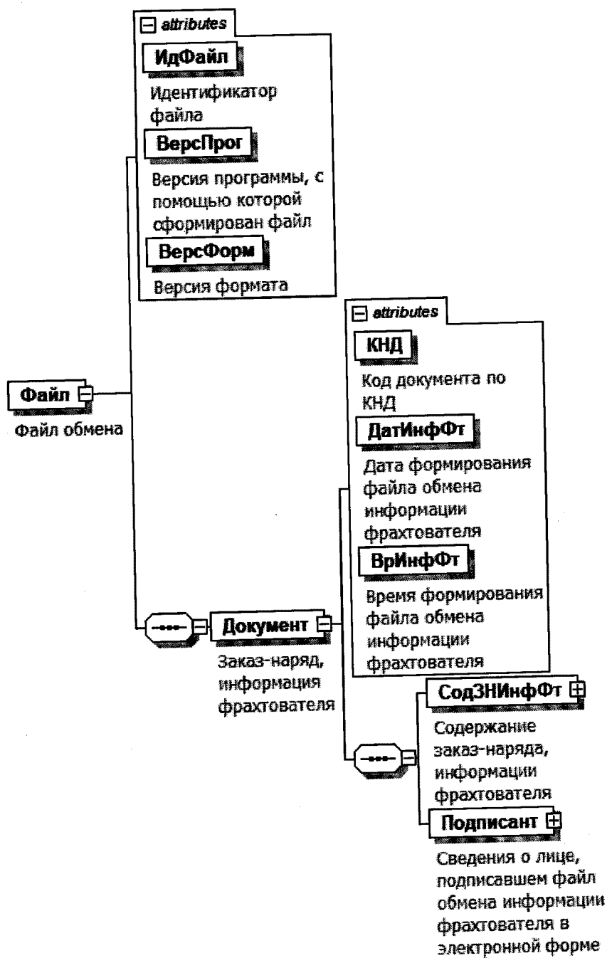
Рисунок 1. Диаграмма структуры файла обмена
