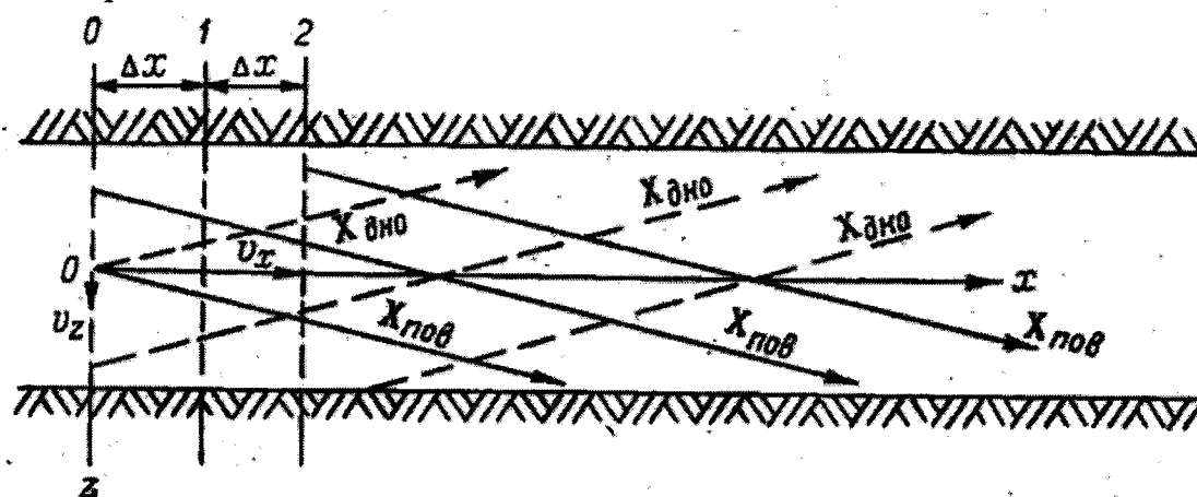
Рис.8. Расположение координатных осей в поверхностном и придонном слоях потока.
