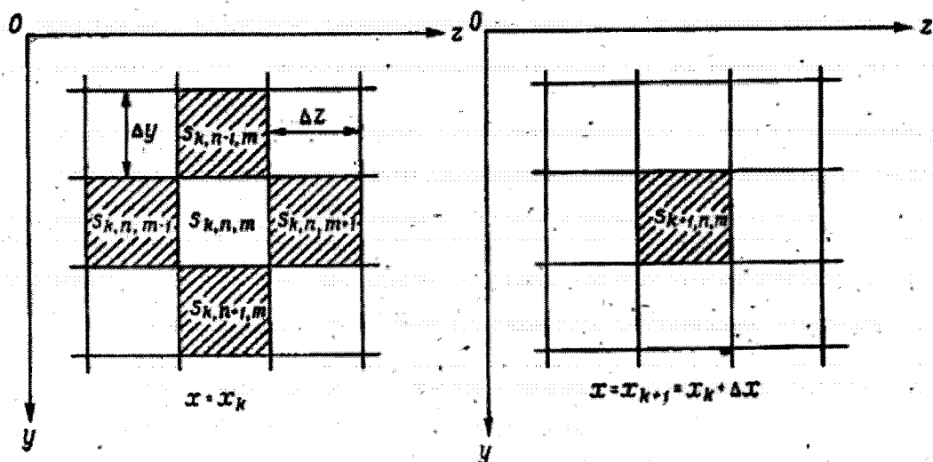
Рис. 6. Сетка к расчету турбулентной диффузии. Пространственная задача.
