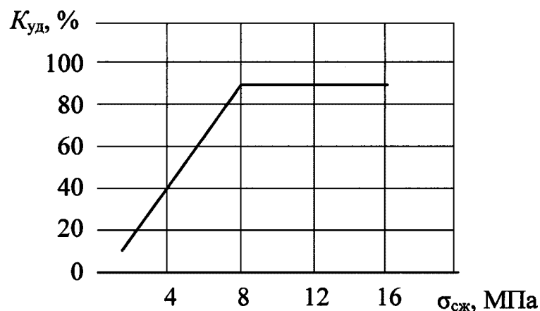
Рис. 1. График зависимости K_{\text{уд}} от \sigma_{\text{сж}} .
