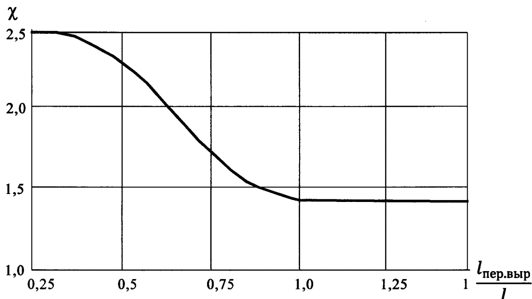
Рис. 11. Номограмма для определения \chi : l_{\text{пер.выр}} – расстояние от забоя лавы до передовой выработки, м; l – ширина зоны опорного давления, м.
