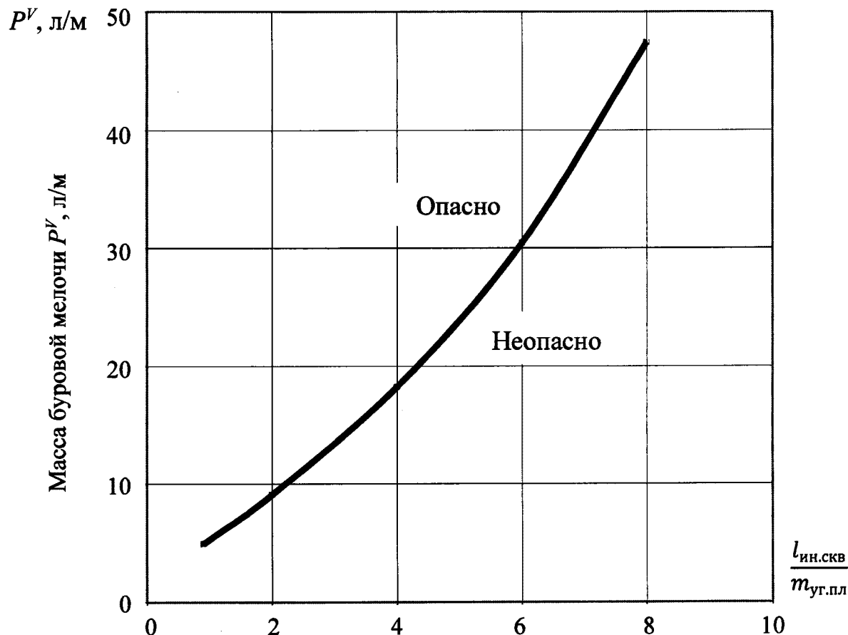
Рис. 5. Номограмма для установления категории «опасно» или «неопасно» участков антрацитовых угольных пластов по выходу буровой мелочи.
